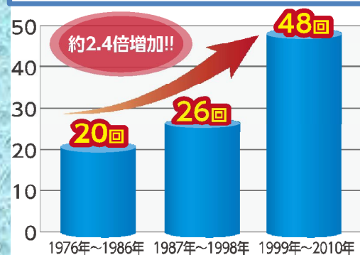
1時間100mm以上の雨の発生回数
