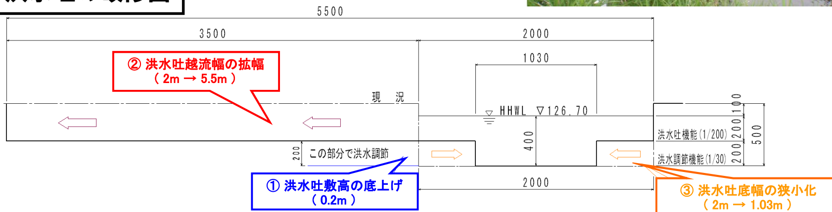
洪水吐の改修図
