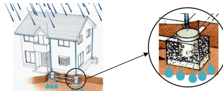
浸透柵のイメージ
