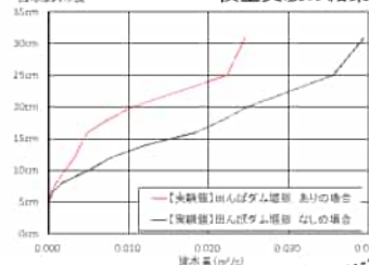
模型実験の結果
