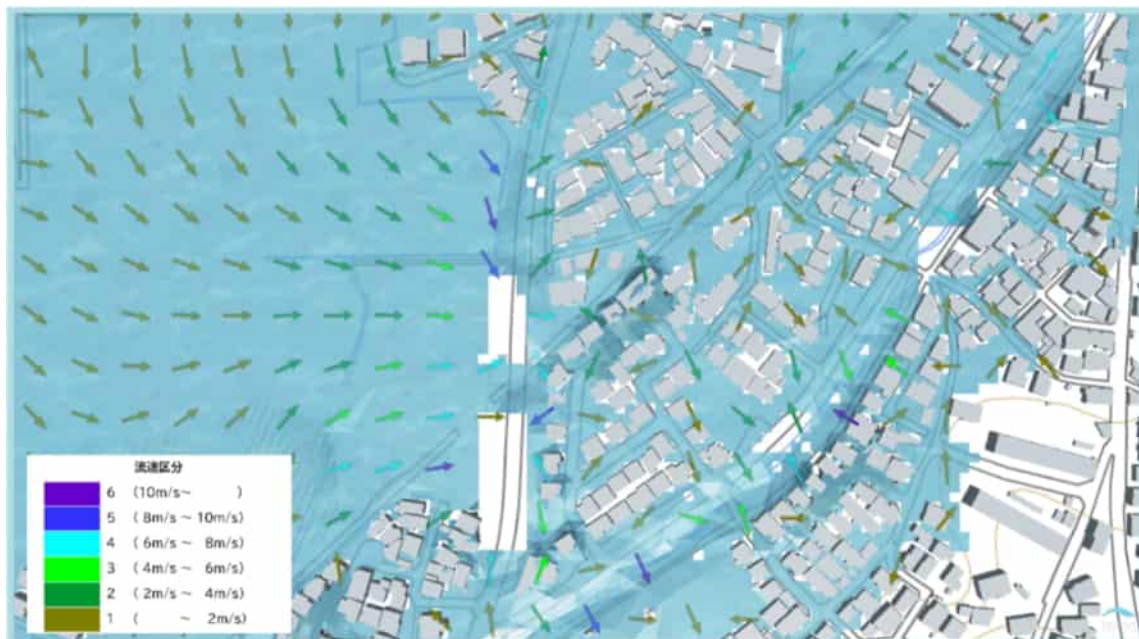
浸水シミュレーションによる流速ベクトル図
