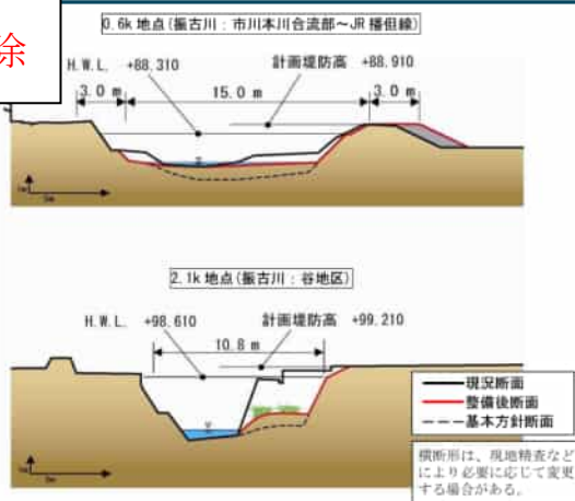
振古川整備横断イメージ
