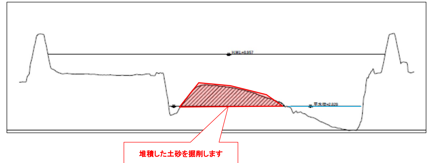
施工状況図
