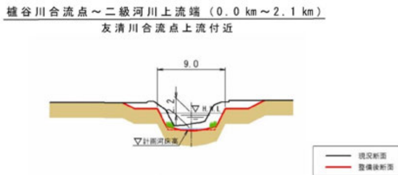
図 26 友清川整備断面イメージ
