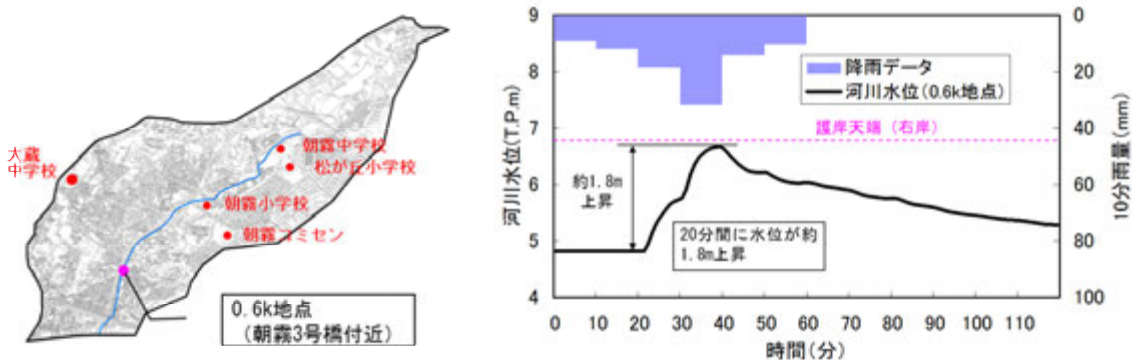
朝霧川0.6k地点の水位上昇速度
