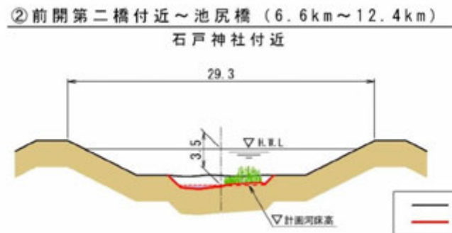
図 24 伊川整備断面イメージ
