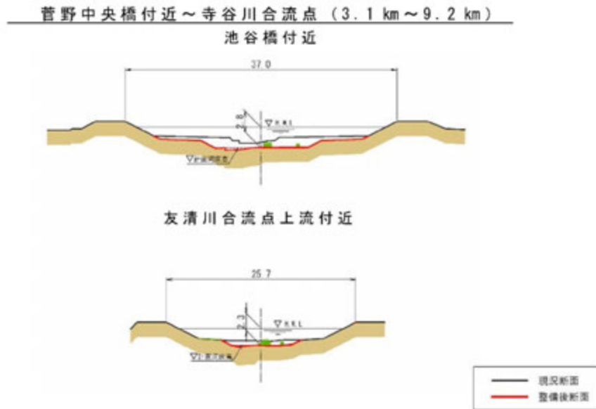
図 25 櫛谷川整備断面イメージ
