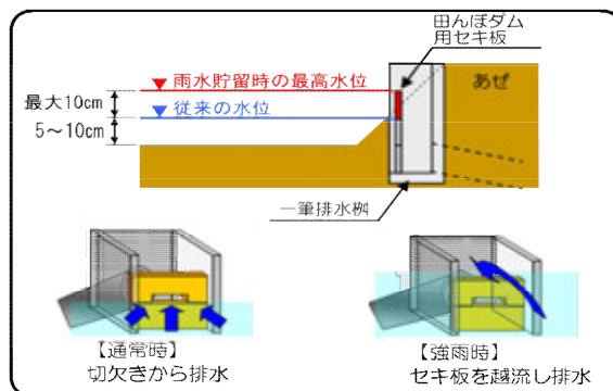
図 34 田んぼダムセキ板
