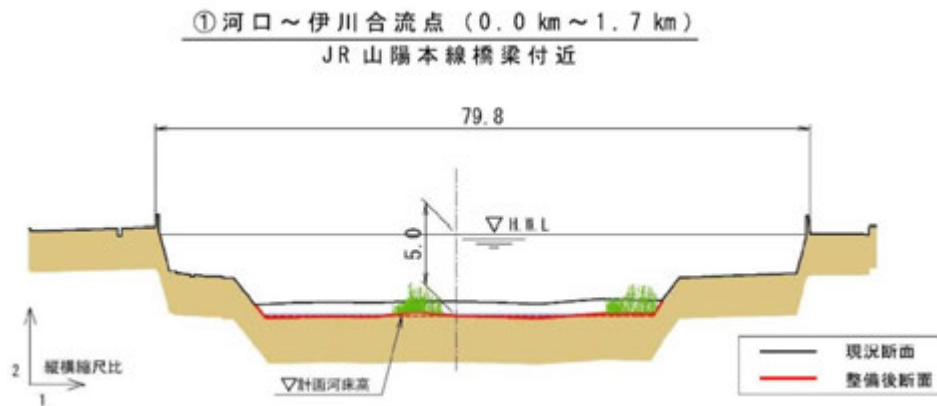
図 23 明石川整備断面イメージ
