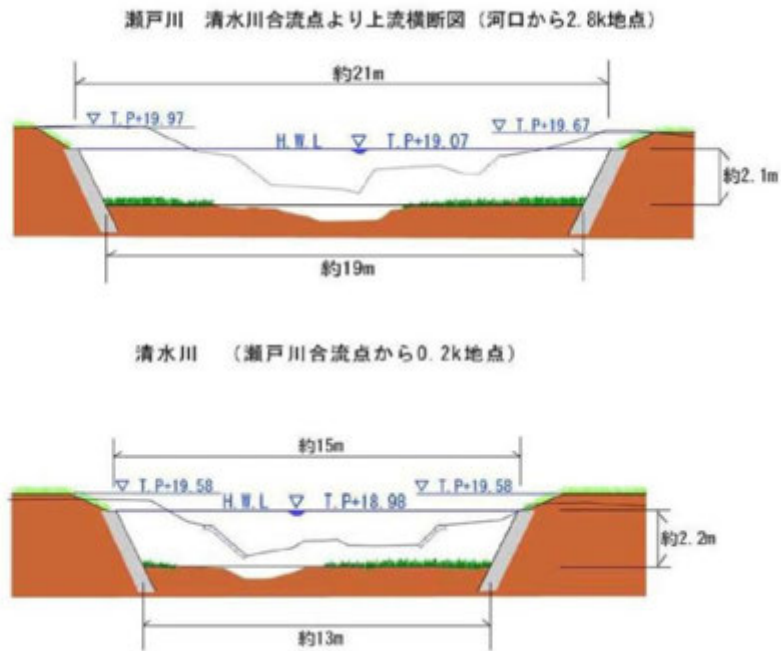
図 28 瀬戸川水系整備イメージ
