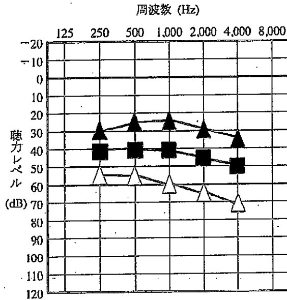
図1-B 音場における聴覚閾値 補聴器非装用時 (△), 補聴器装用時 (補聴器 1: ■, 補聴器 2: ▲) ファンクショナルゲイン (dB) = 補聴器非装用時閾値 - 補聴器装用時閾値
