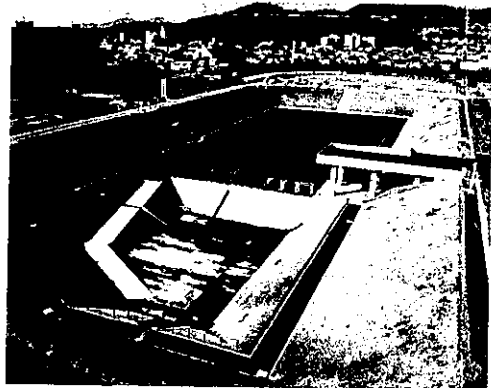
姫路競馬場内に整備された船場川の洪水調節池。25にプール約400個分という県下最大の規模で、平常時にはサッカー場として利用できます
