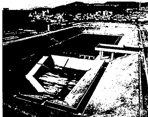
姫路競馬場内に整備された船場川の洪水調節池。25haプール約400個分という県下最大の規模で、平常時にはサッカー場として利用できます
