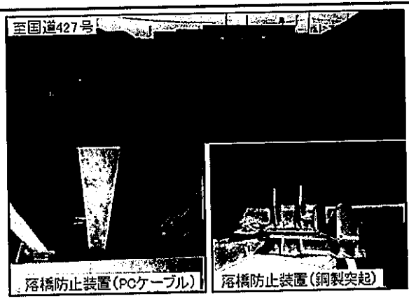
県道西脇口吉川神戸線(春日橋)/西脇市
