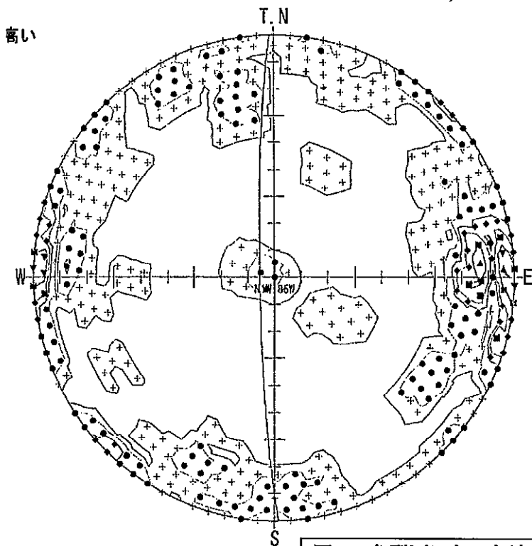
図9 亀裂面にたてた法線と球面との交点 亀裂面が南北方向でやや西に傾く面が多いことが読み取れる
