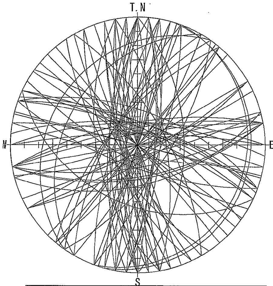
図8 亀裂の方向を示すステレオネット 南北、東西方向で高角の亀裂が多い
