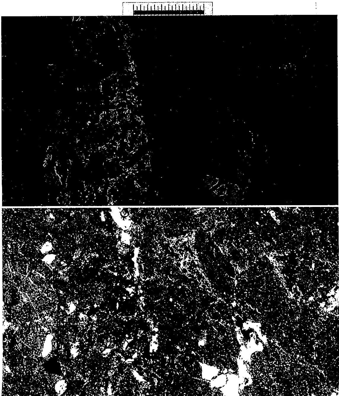
写真6 低倍率の観察（上：平行ニコル，下：クロスニコル，スケールの全長は1mm）
