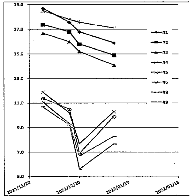
図 3 0 梨ヶ原川, 安室川, および千種川とそれに接する井戸の水温の時間変化
