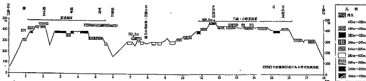
図3 上郡高原の地形面と各面の高度（東西方向断面）
