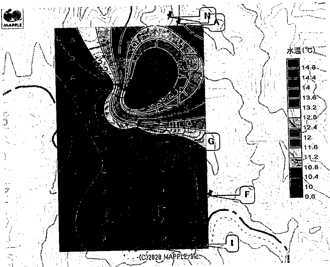
図19 2022年1月30日の地下水温等値線図
