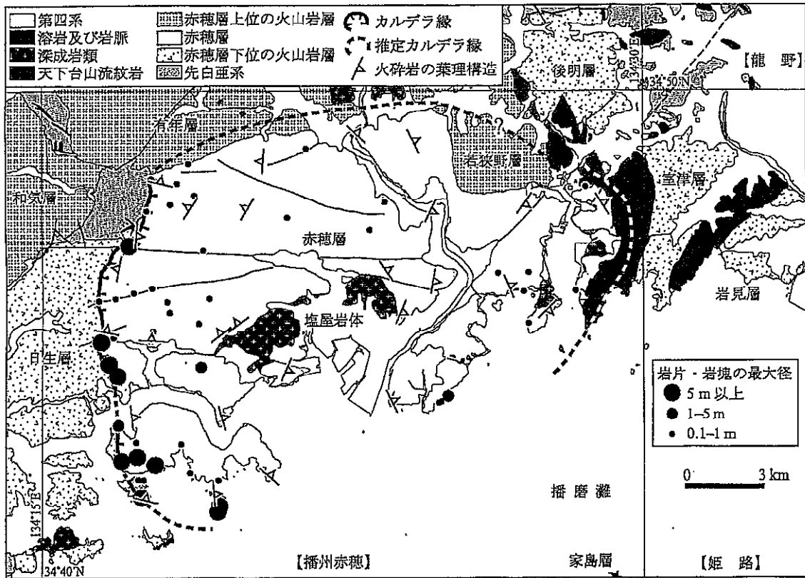
図4 播州赤穂地域の地質の概要
