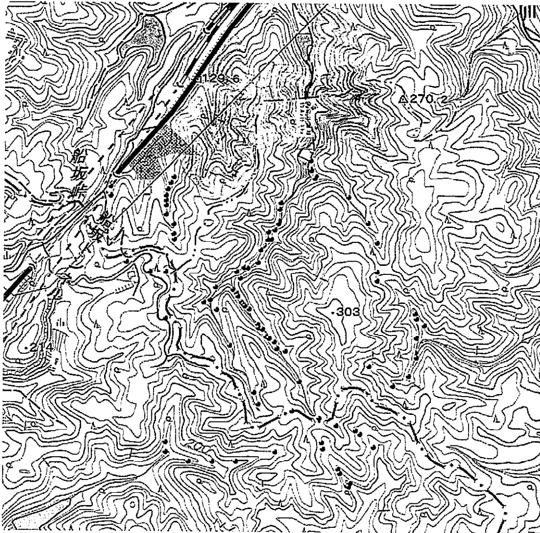
図 7 有年層溶結凝灰岩の断層・亀裂の調査地点
