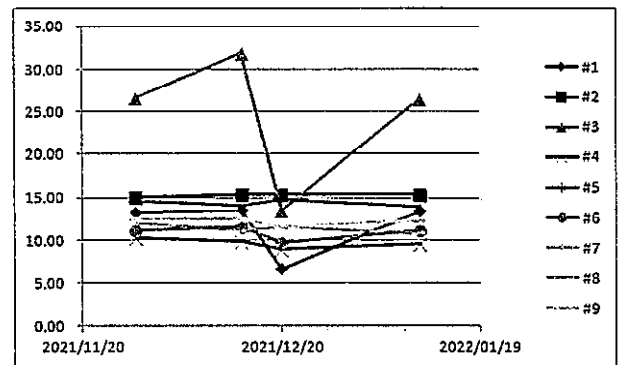
図 3 2 梨ヶ原川, 安室川, および千種川とそれに接する井戸の電気伝導度の時間変化
