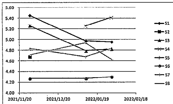
図 3 1 論気谷の河川とため池の電気伝導度の時間変化
