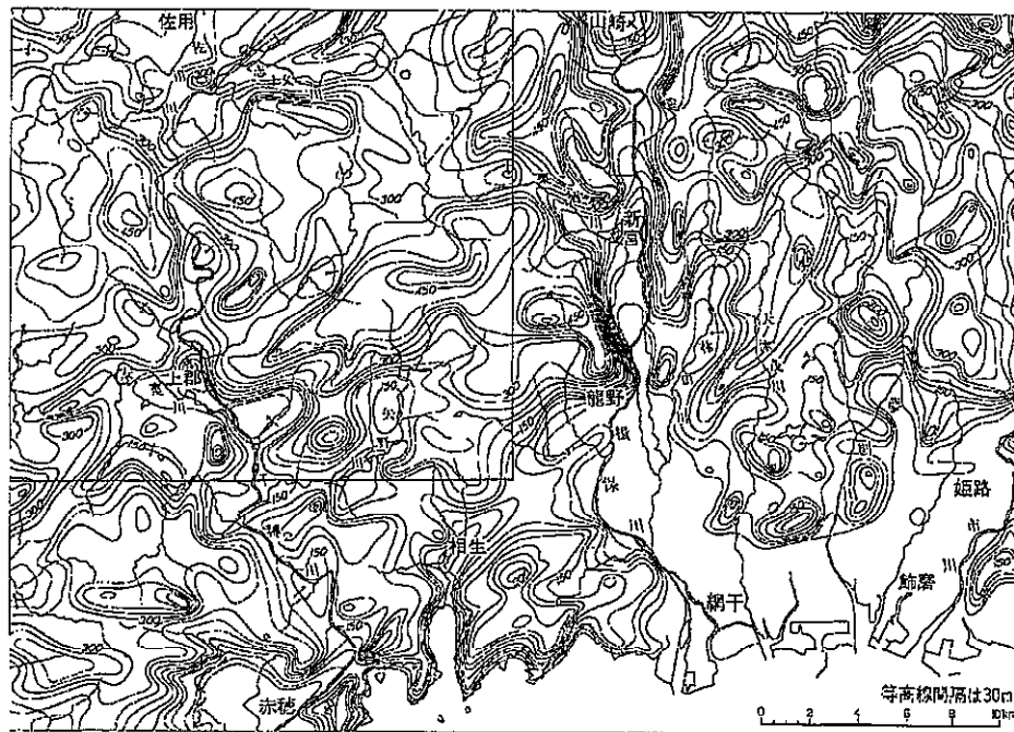
図2 龍野市付近の接峰面図：（猪木・弘原海,1980）より引用 四角の囲みは上郡図幅の範囲
