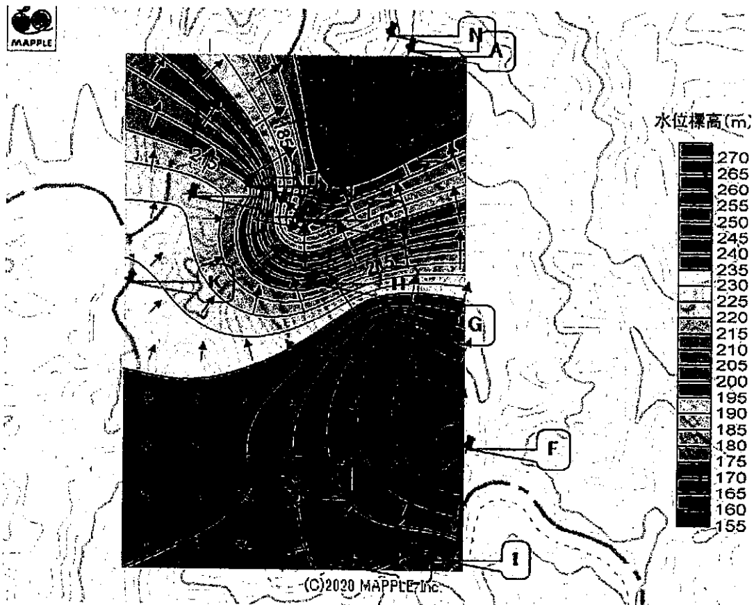
図1 5 2022年2月14日のボーリング水位等高線図
