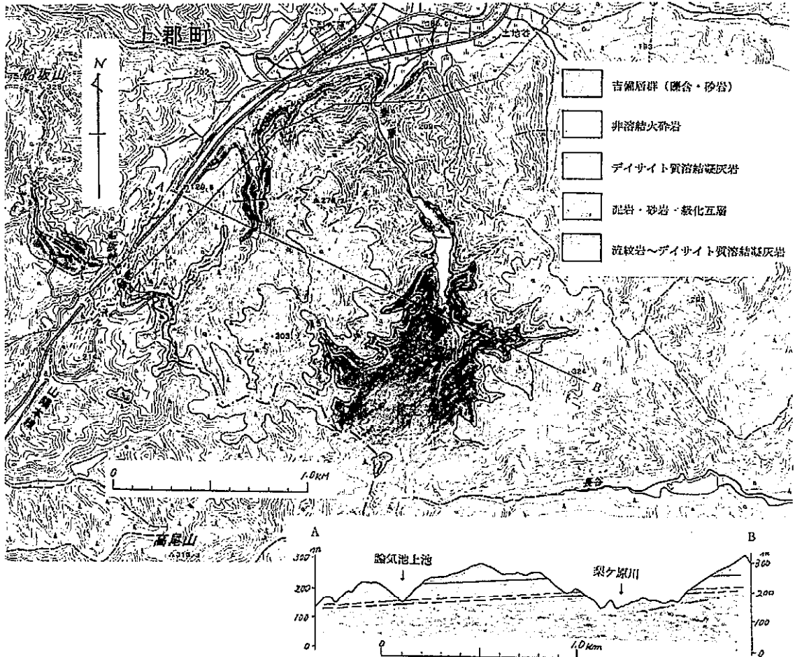
図6 論気川および梨ヶ原流域の地質図及び断面図
