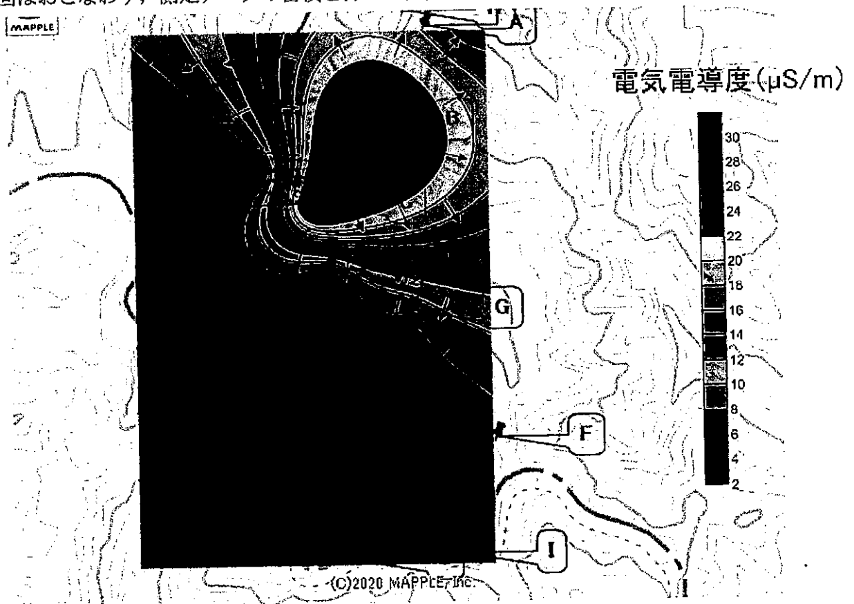
図 2 3 2021 年 12 月 13 日の電気伝導度の等値線図
