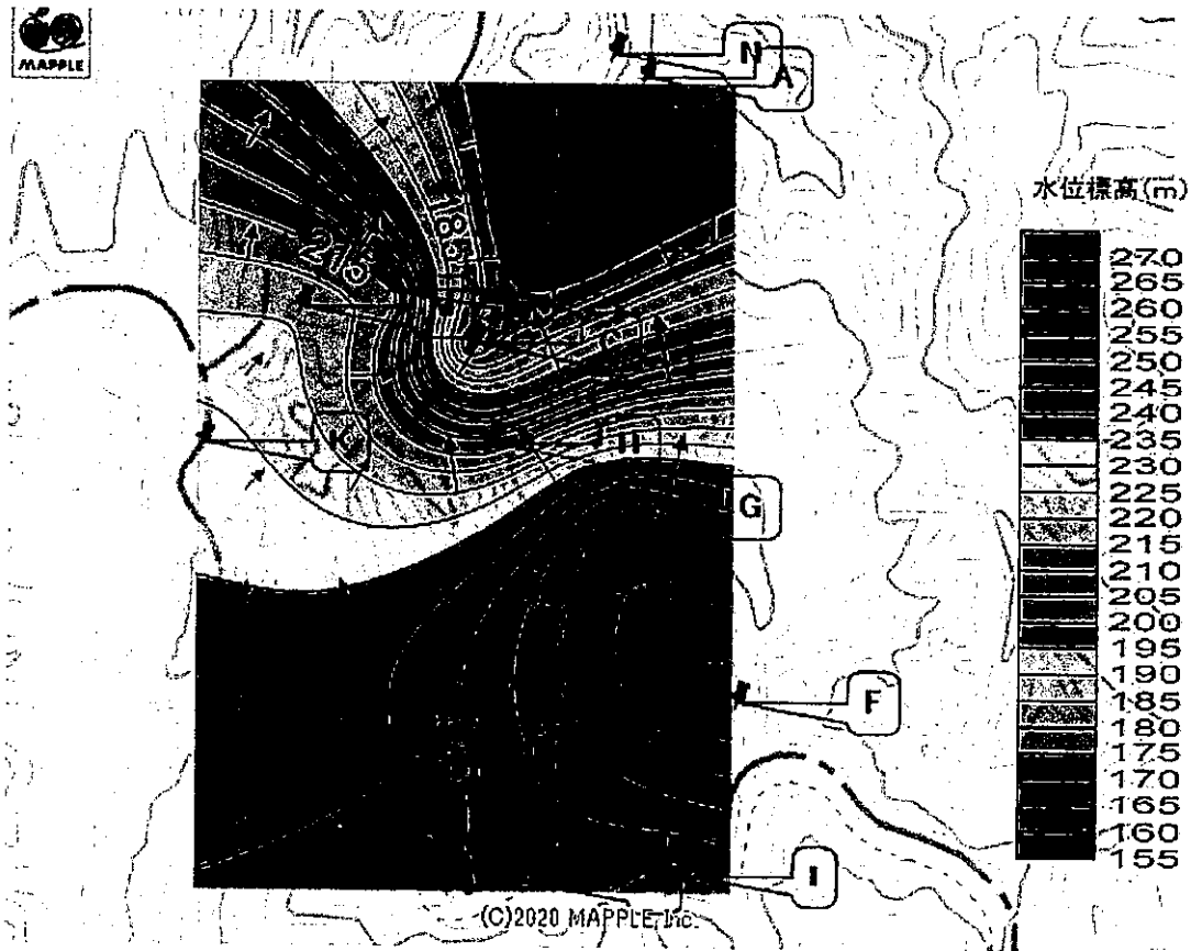
図1 4 2022年1月30日のボーリング水位等高線図
