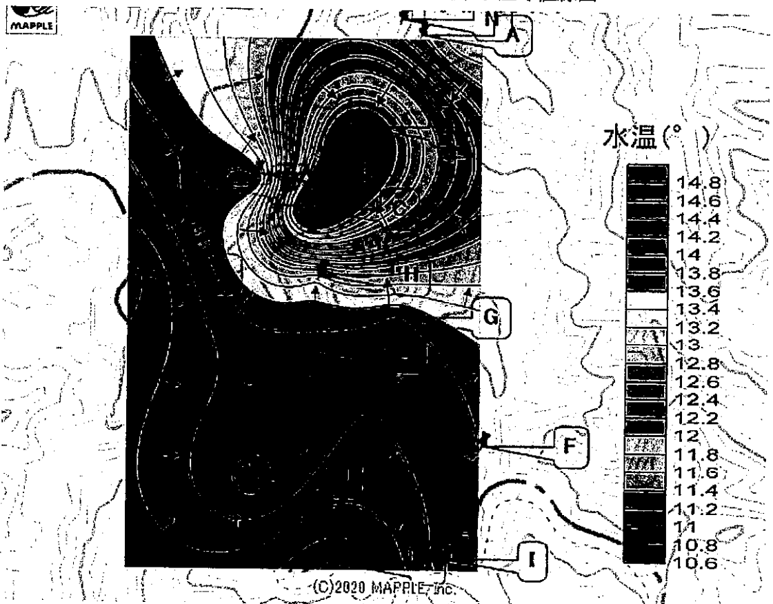
図 1 8 2022 年 1 月 10 日の地下水温等値線図
