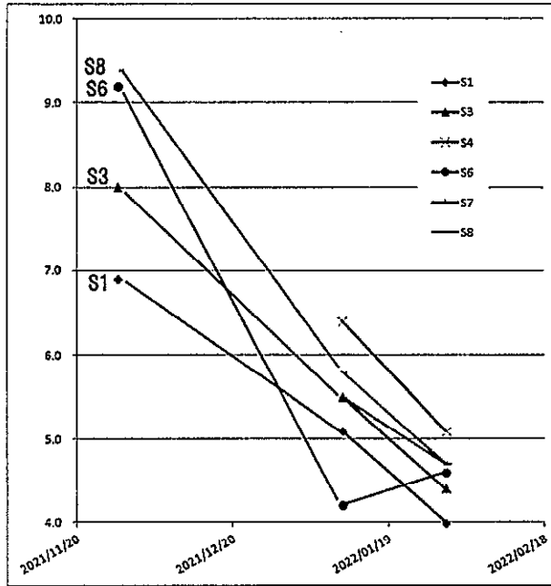
図 2 9 論気谷の河川とため池の水温の時間変化
