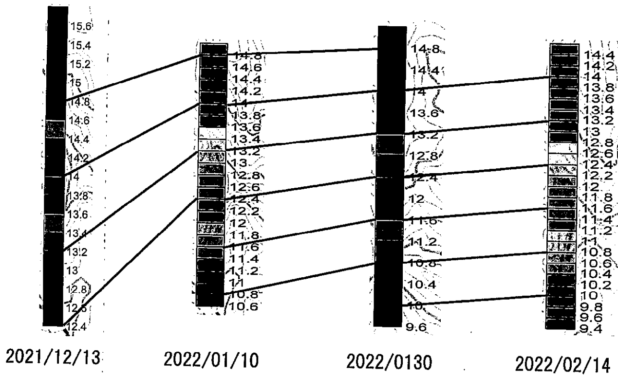
図 2 1 地下水温等値線図の段彩区分の比較
