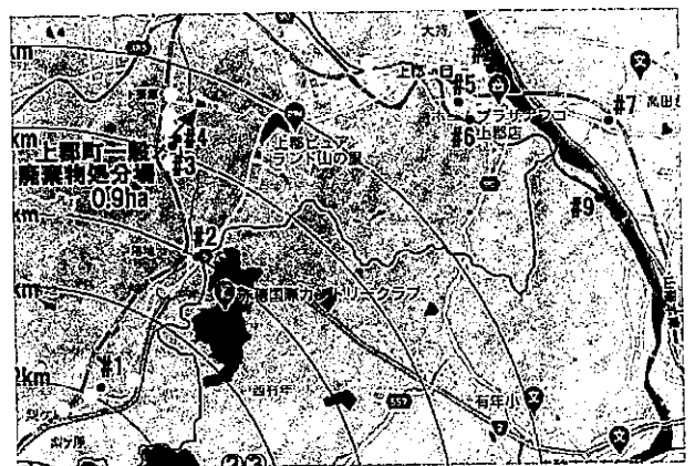
図 2 8 井戸水と河川水の調査地点
