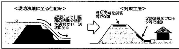
堤防強化対策のイメージ（堤防天端の保護、堤防法尻の補強）
