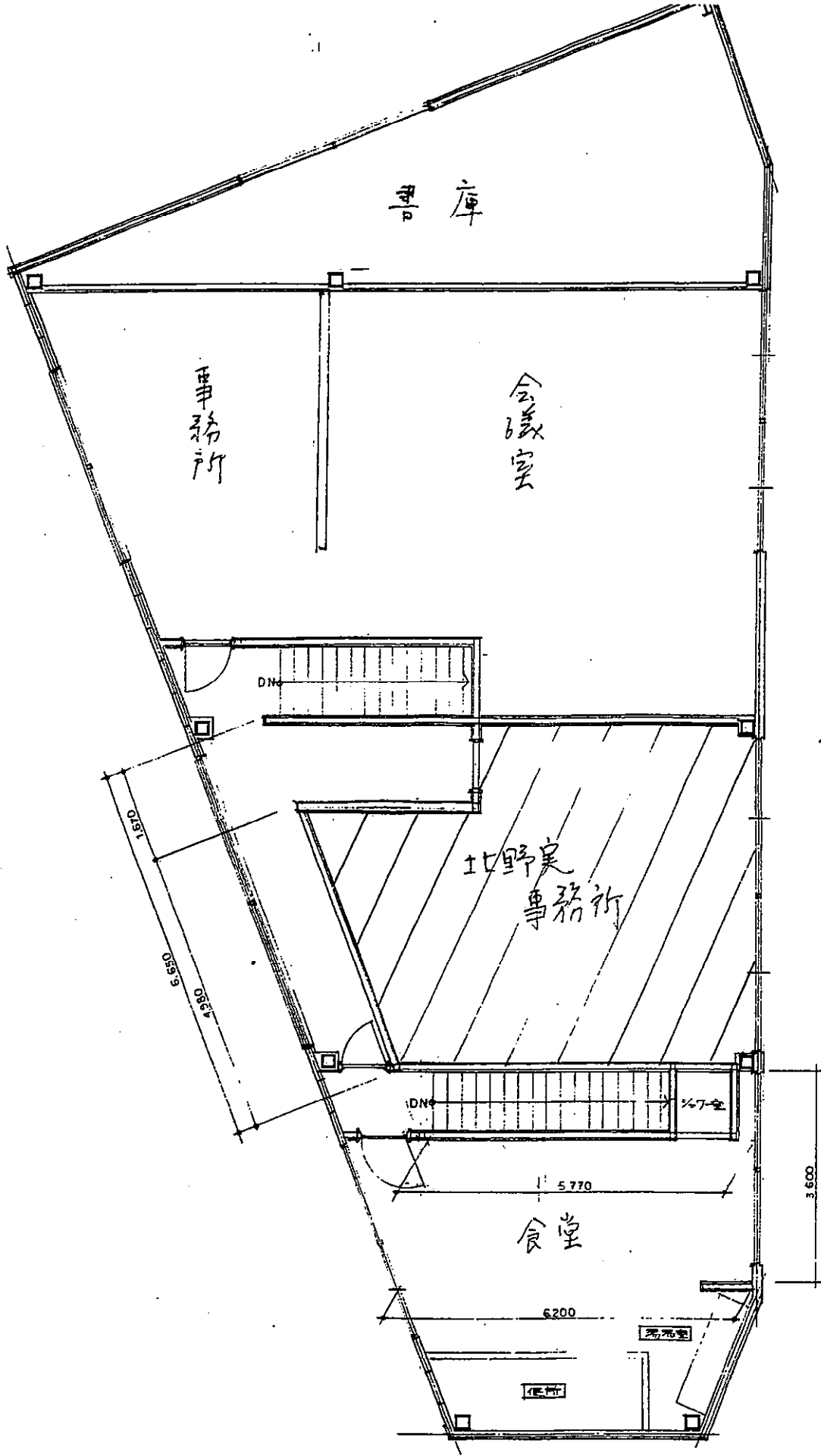
2階平面図
