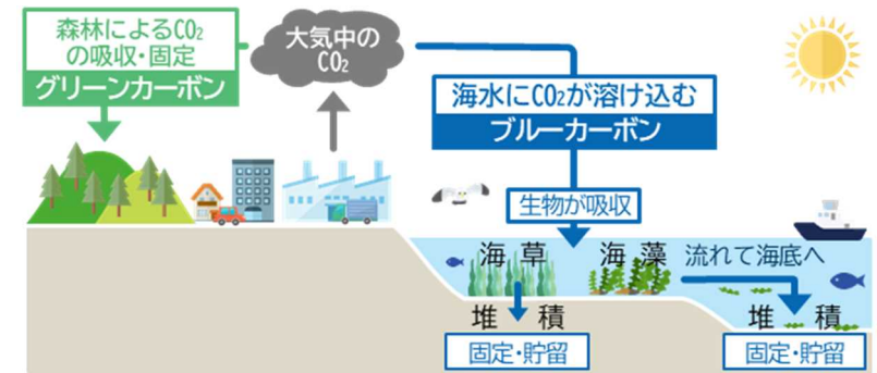
炭素吸収の流れ
