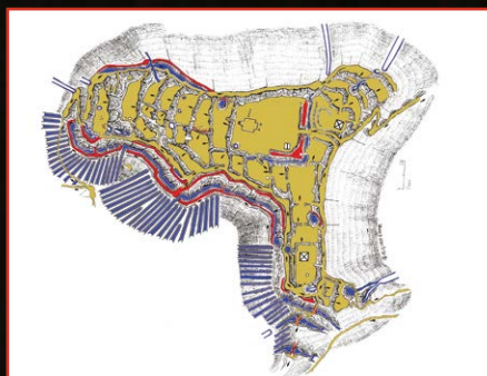
篠ノ丸城測量図
