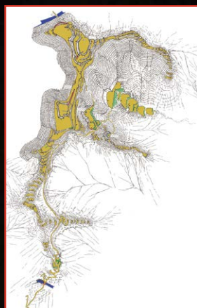
白旗城測量図
