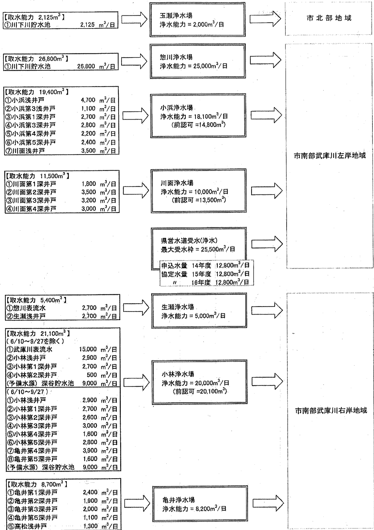
宝塚市の水道用水系統図
