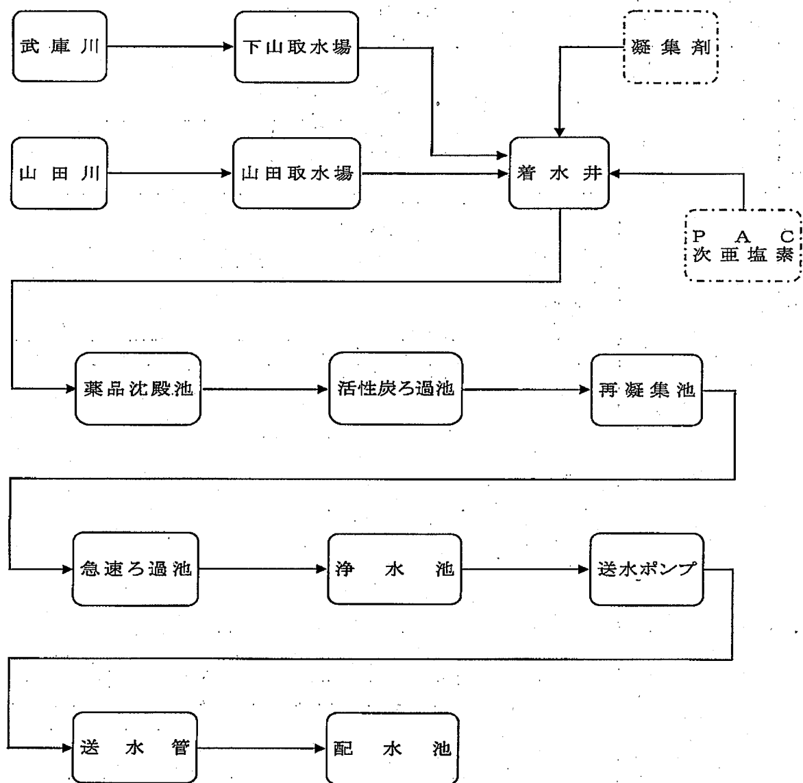
三田市の古城浄水場フロー図
