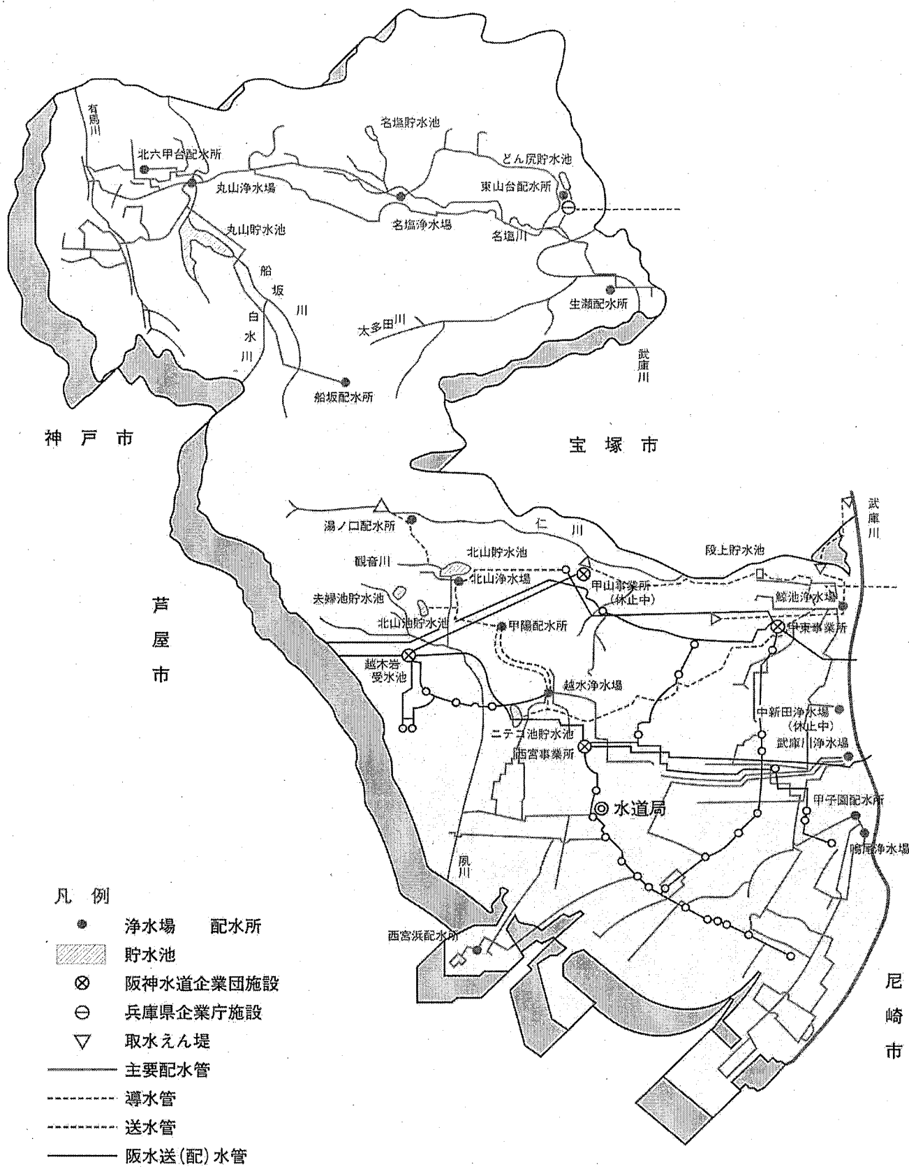
西宮市の水道施設位置図
