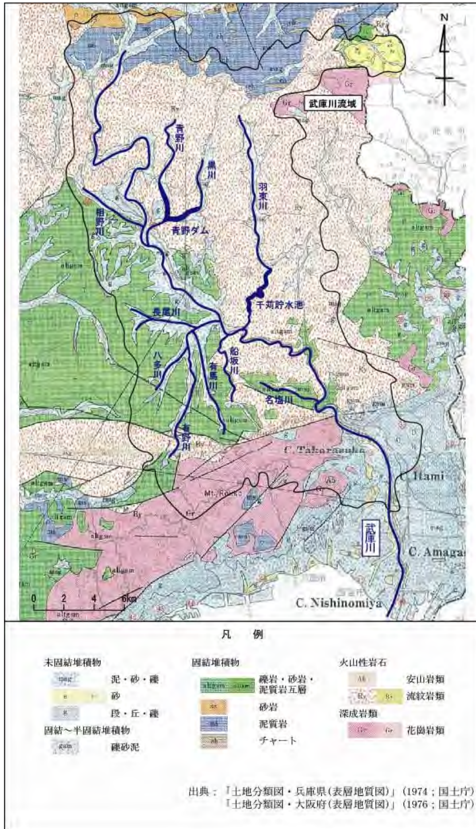
図 1.3.3 武庫川流域の表層地質図（出典：土地分類図）
