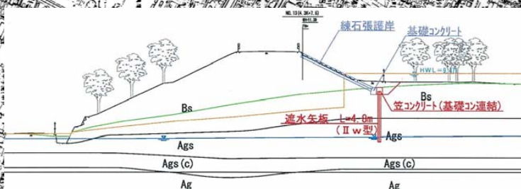
H21堤防補強工事 標準断面図
