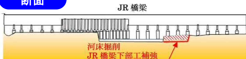
断面
