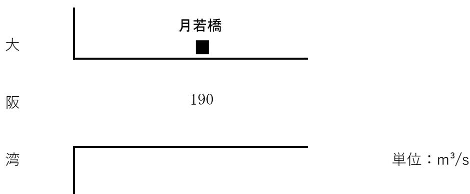
芦屋川計画高水流量図
