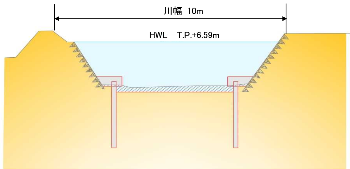
計画横断面図
