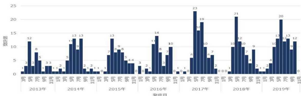
図1. 2013年3月4日以降に届出られたSFTS症例の発症時期 (n=484, 2019年11月27日現在) ※届出対象となる日時以前の発症例8例を除く (SFTSは2013年3月4日に感染症法で全数把握対象疾患である4類感染症に指定された)
