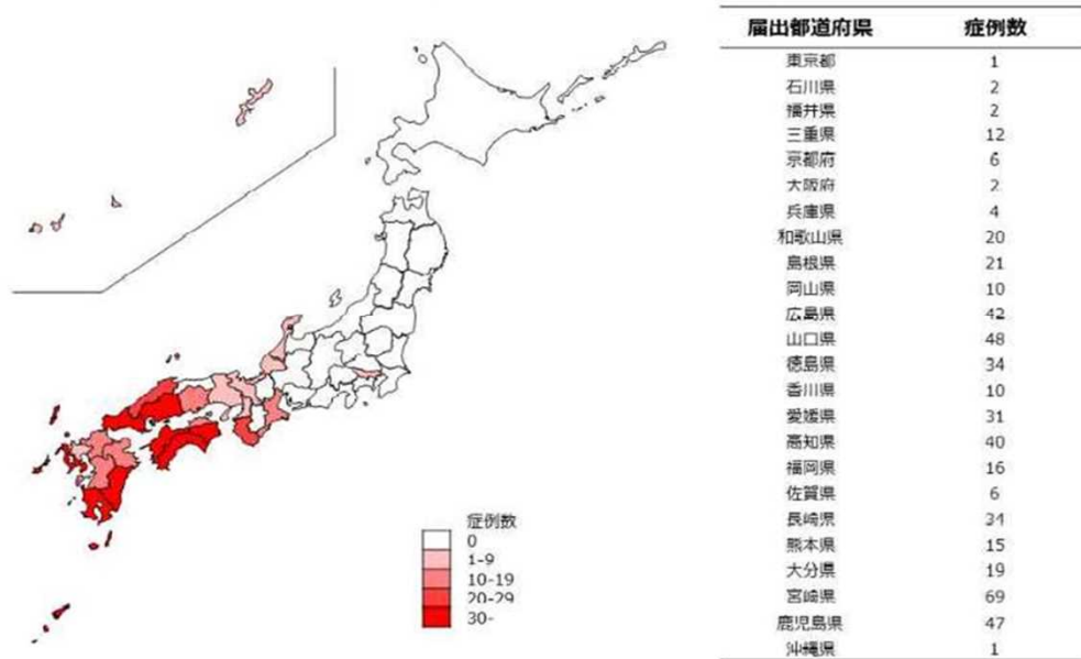
図2. SFTS症例の届出地域（n=492, 2019年11月27日現在）
