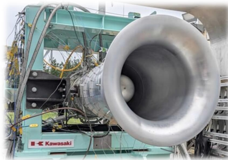
水素航空機用エンジンの試験機 (写真提供:川崎重工業株式会社)
