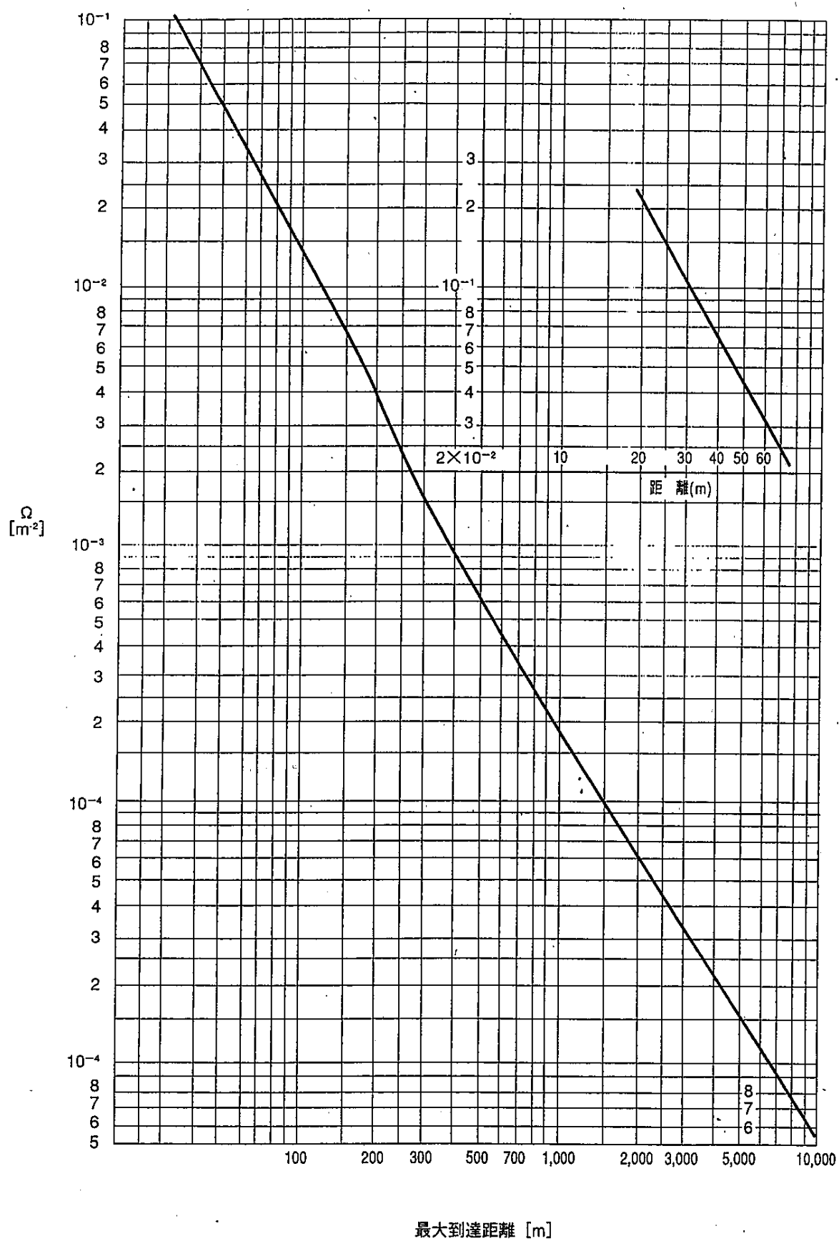
図2 連続発生源からの最大到達距離 (点源高さ h=0.5 m、気象条件：中立)
