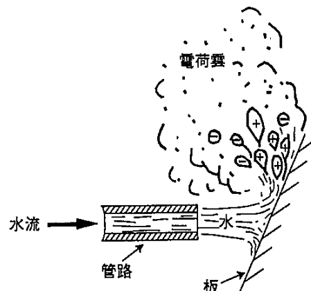
図1 絶縁性液体の管壁からの剥離による帯電
