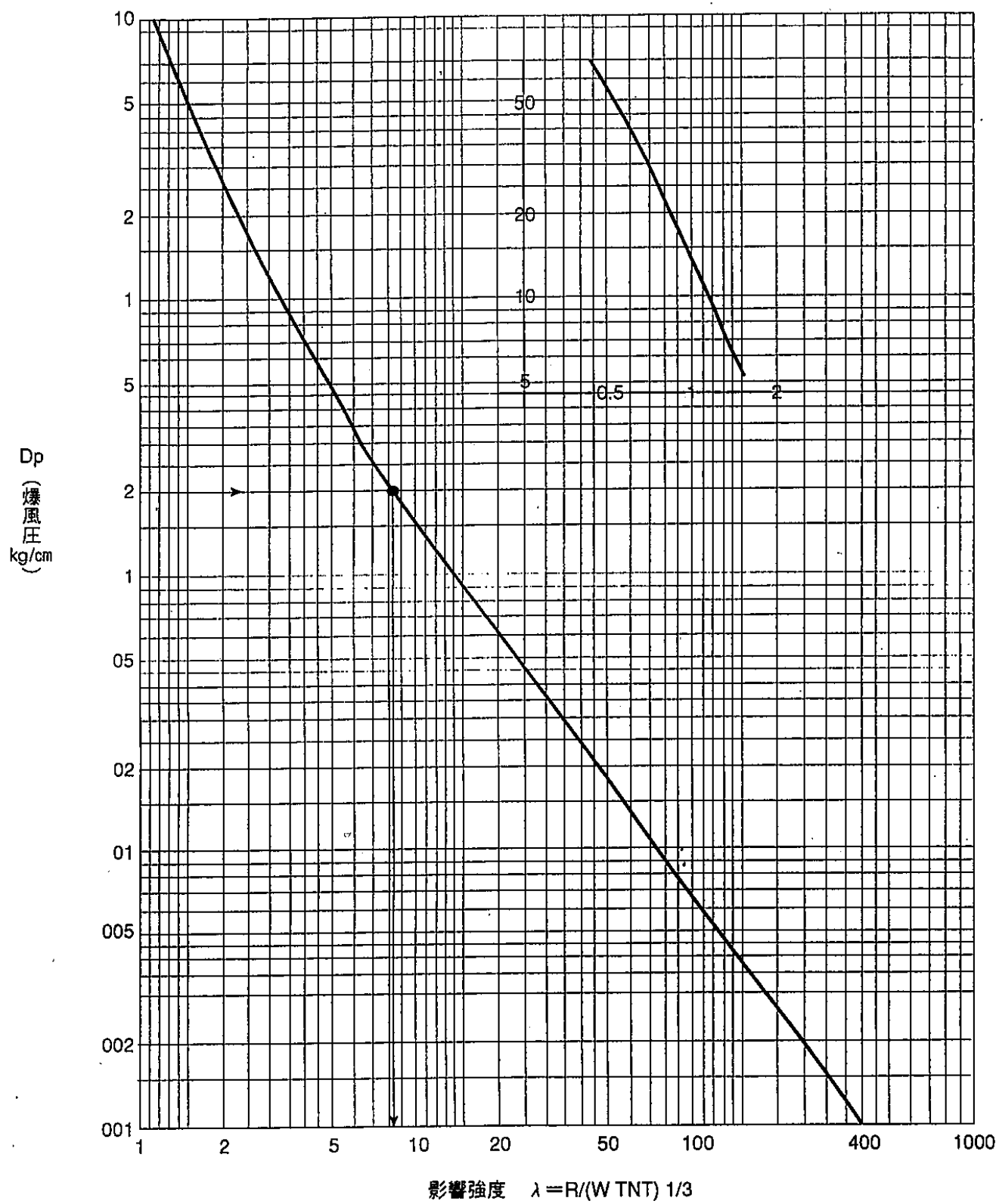
図1 爆風圧対影響強度に関する曲線
