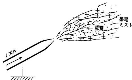
図5 噴霧帯電による放電
