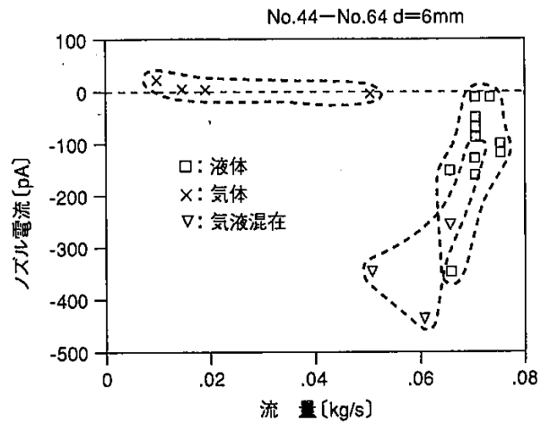
図8 ノズル電流と噴出条件の関係
