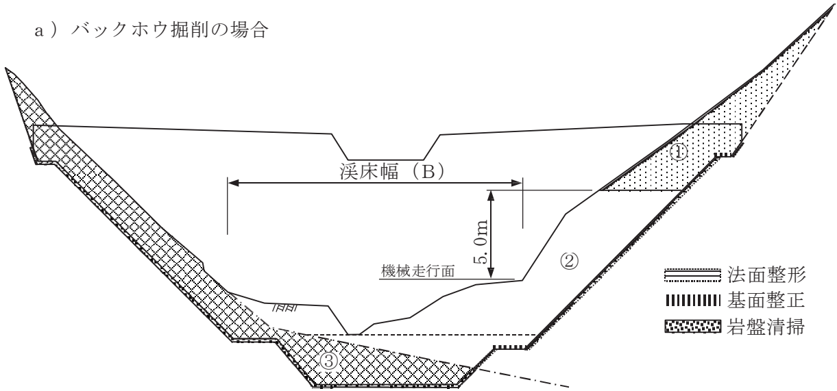
図-1 掘削区分
