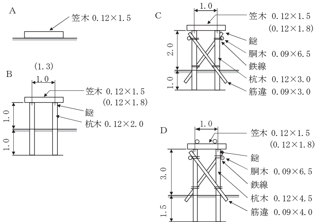
受 枠 の 構 造 図
