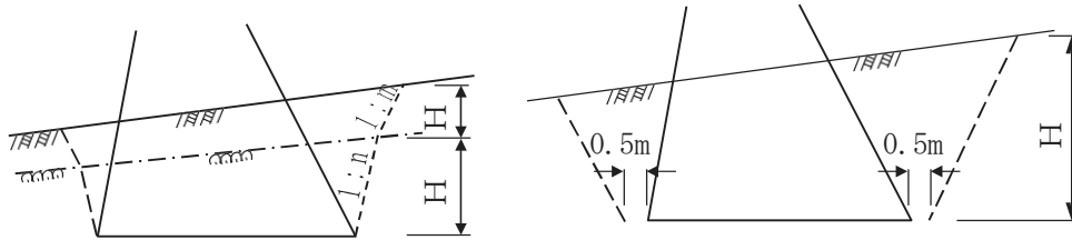
(基礎が岩盤の場合)
