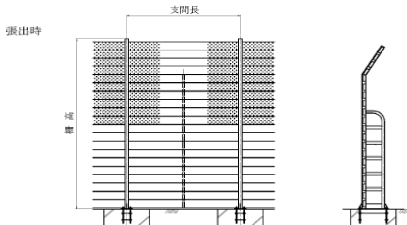
連動型：防雪板全数を同時に張出・収納するタイプ 単動型：防雪板を一枚ごとに張出・収納するタイプ
