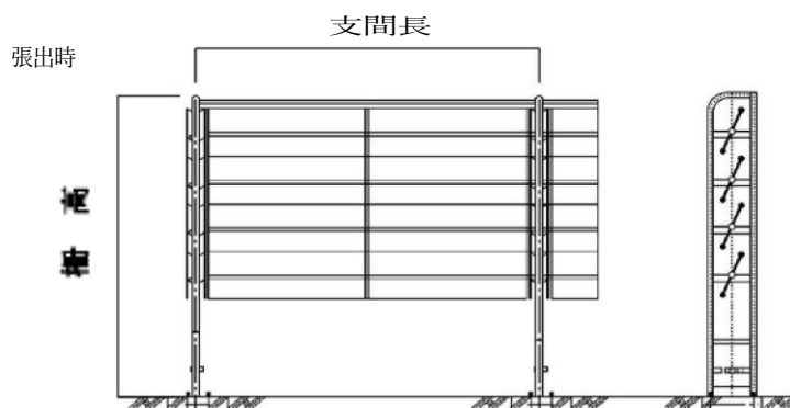
単動型：防雪板を一枚ごとに張出・収納するタイプ
