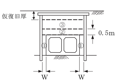
(土留覆工方式)
