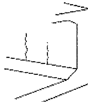
—水和熱（２）—
