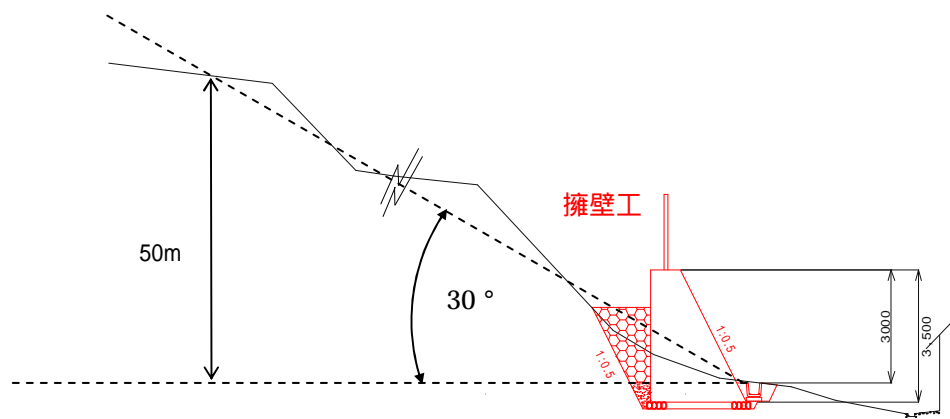
横断図 S = 1:200
