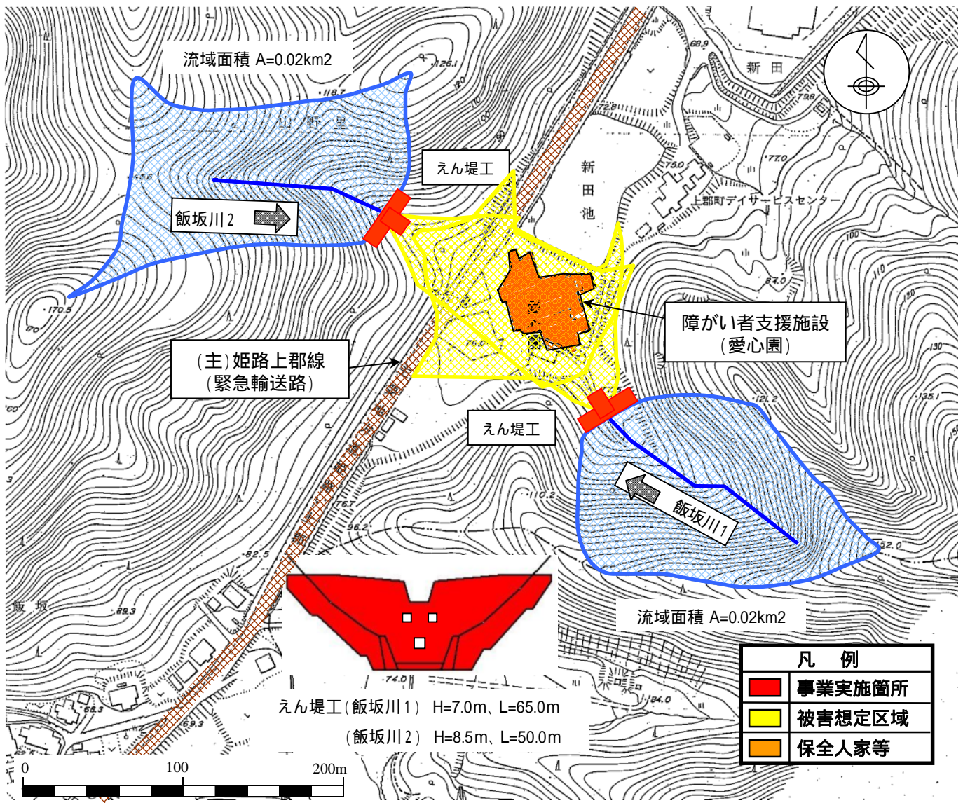
計 画 概 略 図 縮 尺 1 : 3 , 5 0 0
