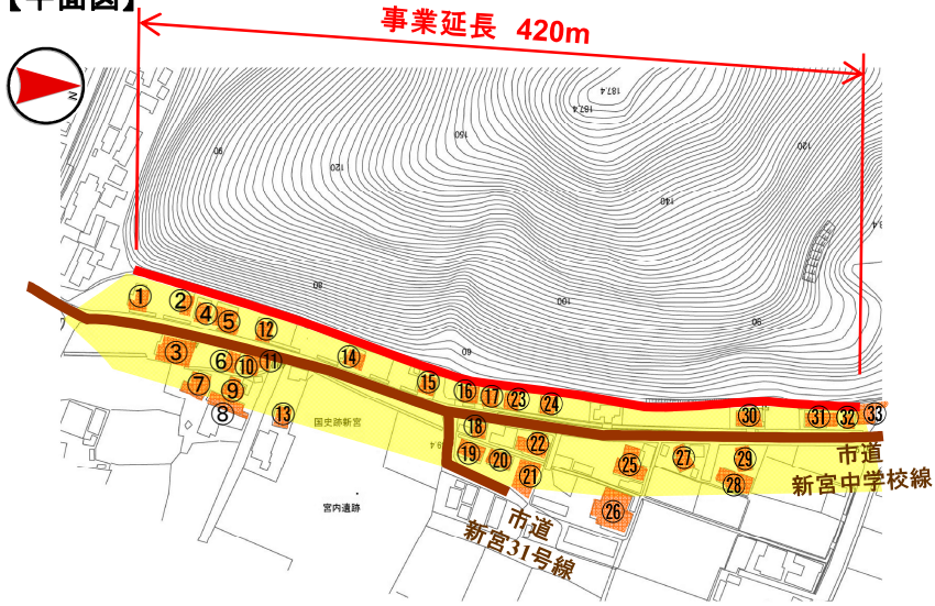
【平面図】
