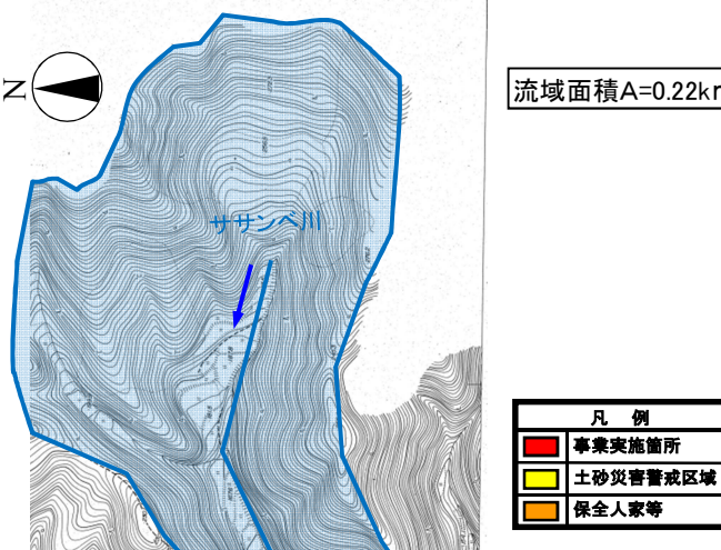
えん堤工
