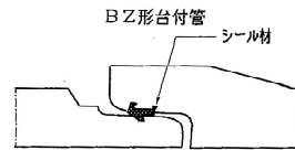
BZ 形台付管・管の受け口に予めシール材が埋込まれた構造 (ガスケットタイプ)
