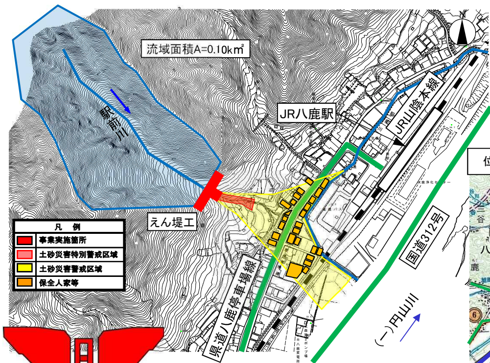
流域面積 A=0.1km 2 事業内容 (全 体) えん堤1基
