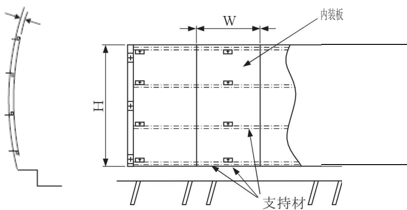
断面図
