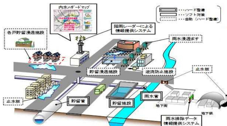
図「下水道(雨水)の整備」の方策事例 (引用：国土交通省ホームページ)
