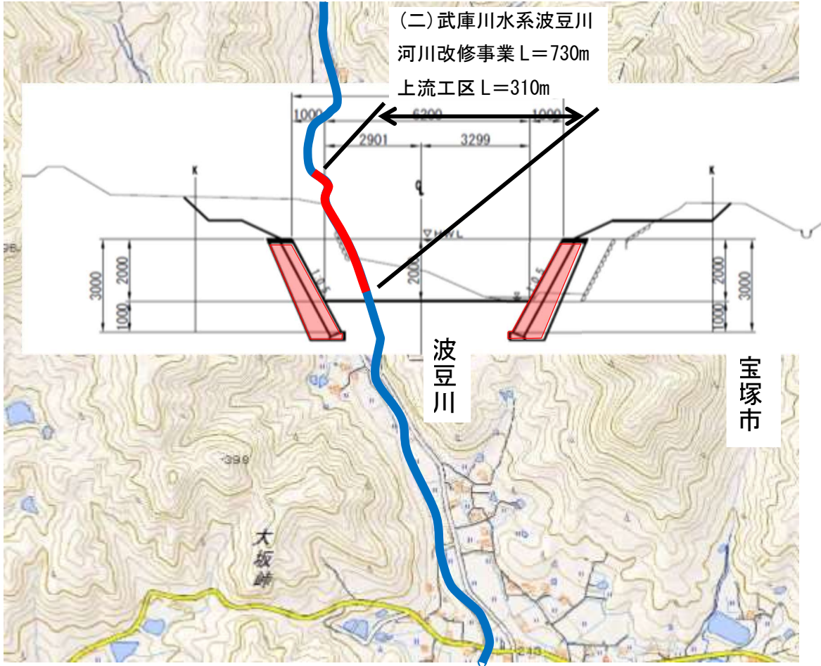
波豆川（上流工区）標準断面図
