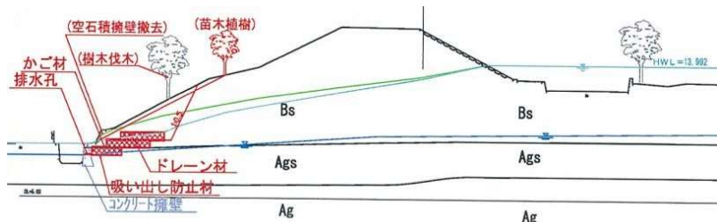
侵食対策(護岸工)標準断面図
