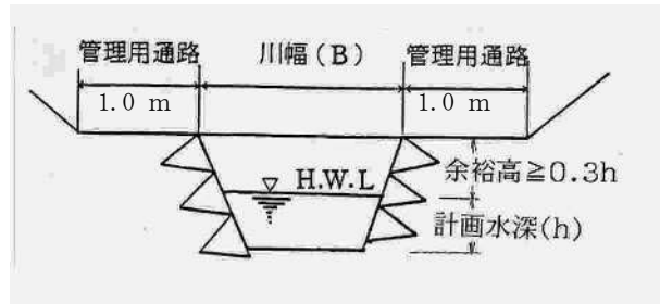
図 3-5 小規模な排水路の余裕高と管理用通路
