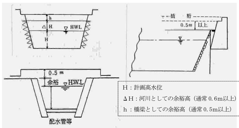
図 3-2 桥梁の桁下高と橋台の構造
