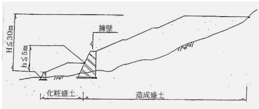
図 1－9 化粧盛土
