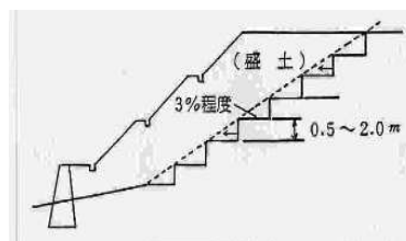
図 1-4 段切り
