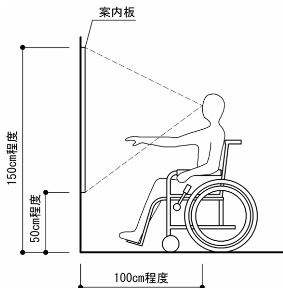
図Ⅲ-13-3 案内板の高さ
