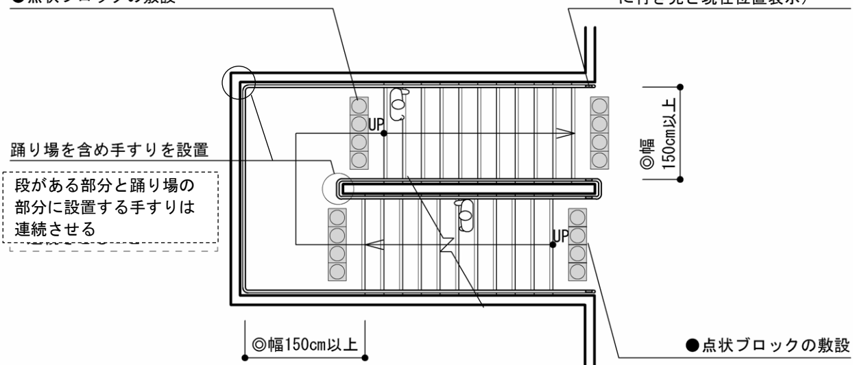
図Ⅲ-4-2 連続手すり
