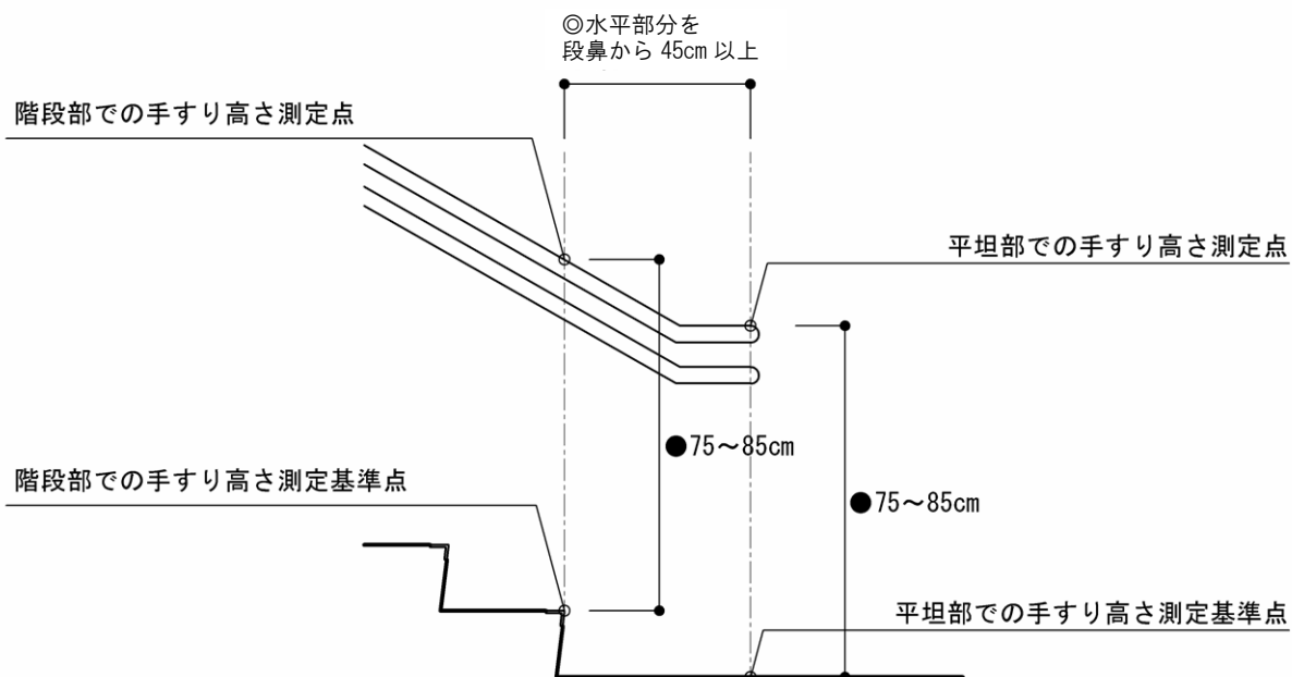
図Ⅲ-4-3 手すりの高さの測り方
