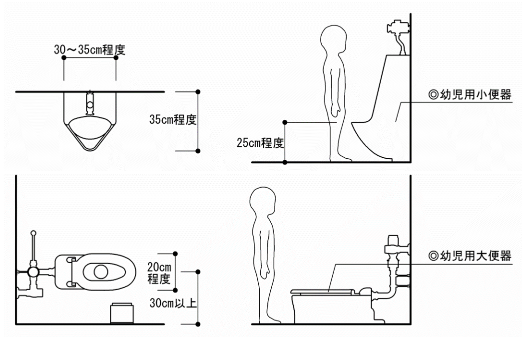
図Ⅲ-7-16 幼児用便器 (大・小)
