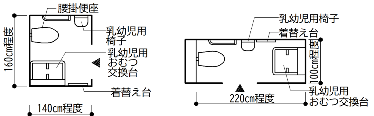
図Ⅲ-7-11 乳幼児用設備を有する便房 (ベビーカーと共に入ることができる寸法)
