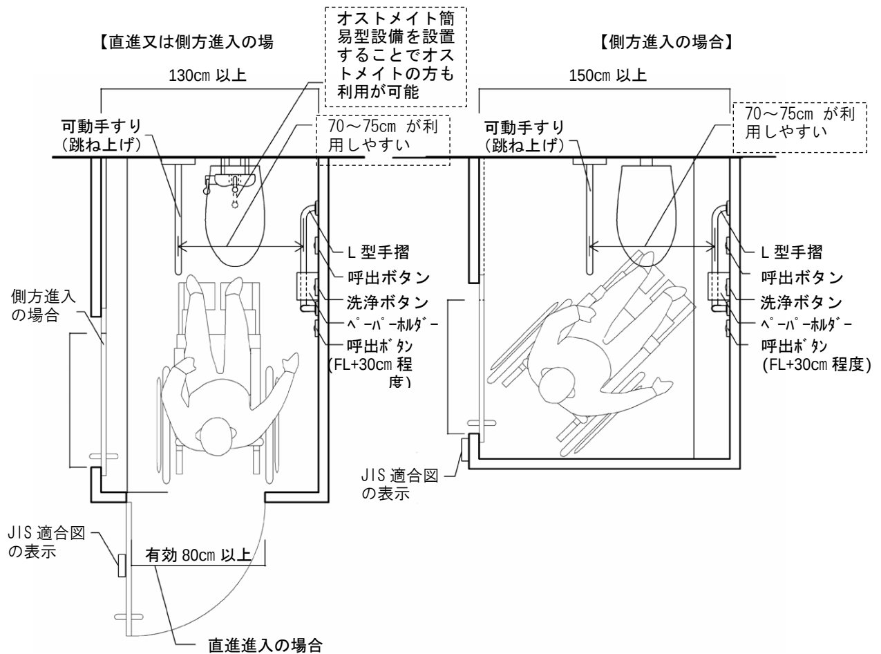
図Ⅲ-7-8 車椅子使用者用簡易型便房（直進又は側方進入の場合） （車椅子使用者利用便房とは別に利用者の分散を図るためその他の便所に整備する場合や、面積や構造に制約がある既存建築物の改善・改修でやむを得ない場合など）
