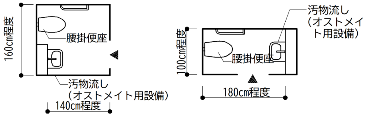
図Ⅲ-7-10 オストメイト用設備を有する便房
