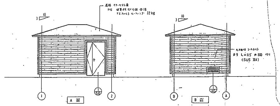
立面図 1/50
