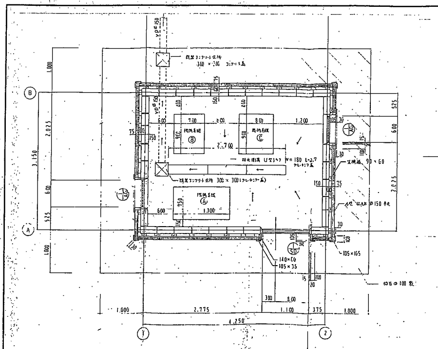
平面図 1/30
