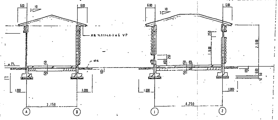
断面図 1/50
