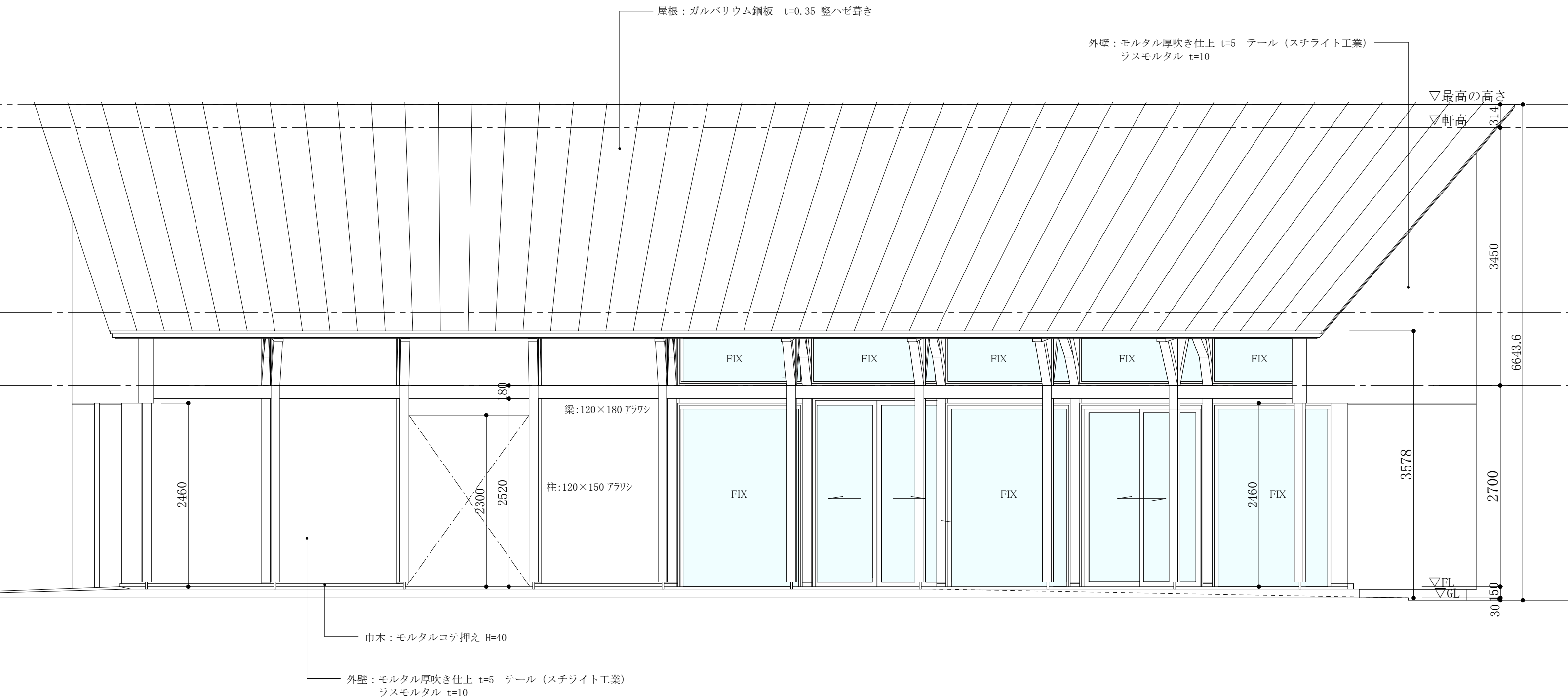
北側立面図
