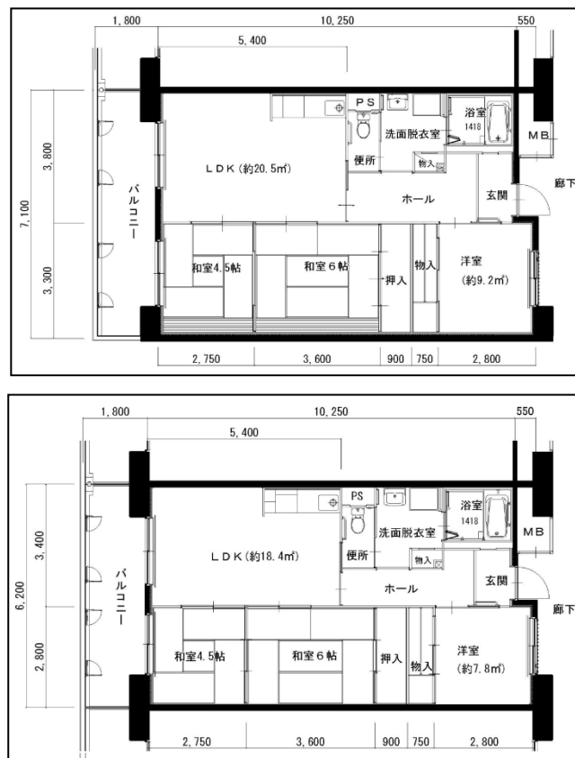
<住戸平面図>
