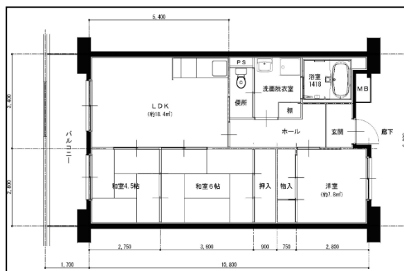
<住戸平面図>
