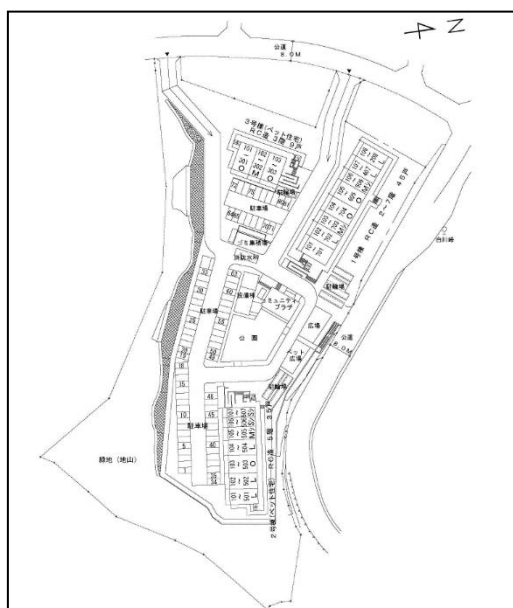
<住棟図>
