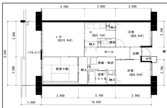
<住戸平面図>
