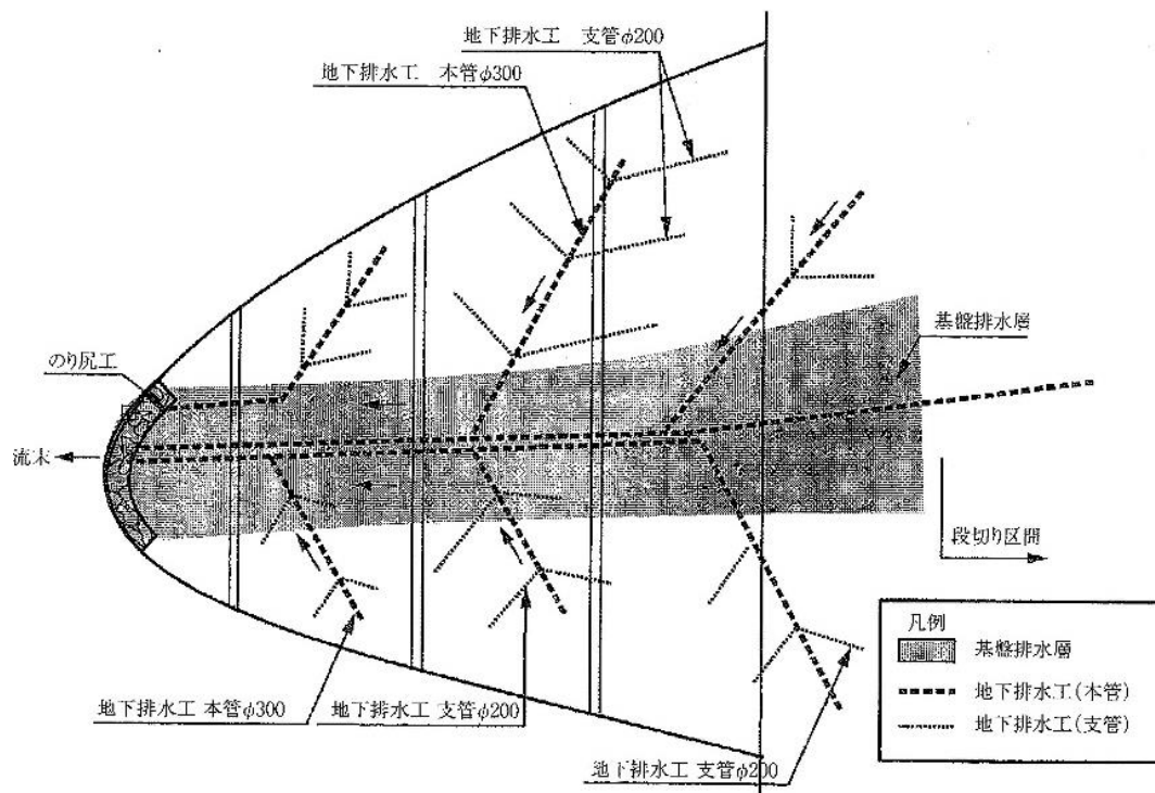
図6-4-4 &lt;盛土内の暗渠排水工及び基盤排水層の設置例&gt;
