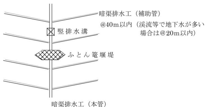
図 6 - 4 - 7 &lt;ふとん箇堰堤の例&gt;
