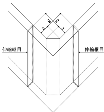
(b) 立体図
