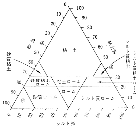
〈図2-4-2〉三角座標による土の分類
