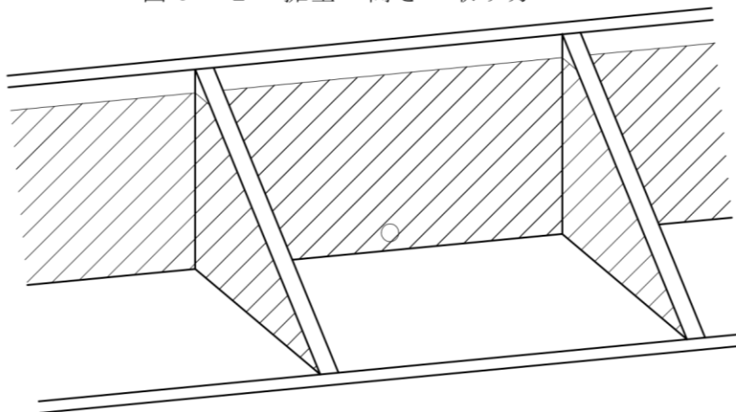
図 5 - 3 控え壁式擁壁の場合の透水マットの取付位置
