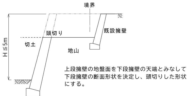
図4-7-2 &lt;上段擁壁等による荷重を考慮した下段の練積み造擁壁の形状&gt;
