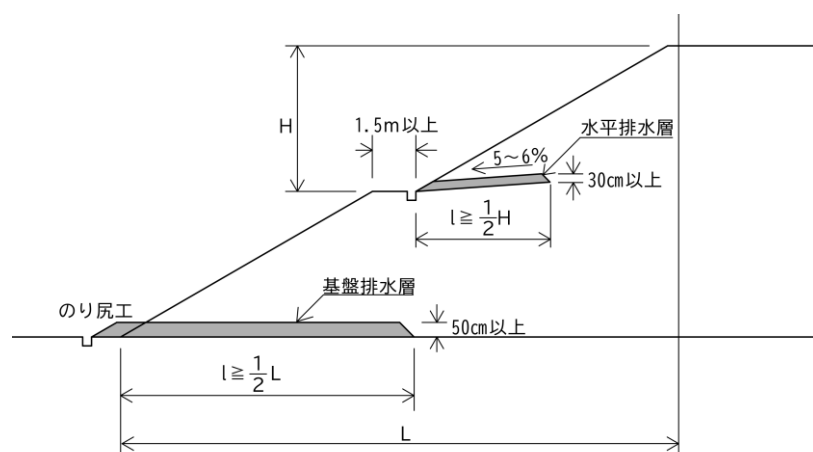
図6-4-5 &lt;基盤排水層及び水平排水層の例&gt;
