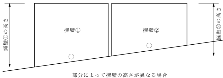
図 5 - 2 擁壁の高さの取り方
