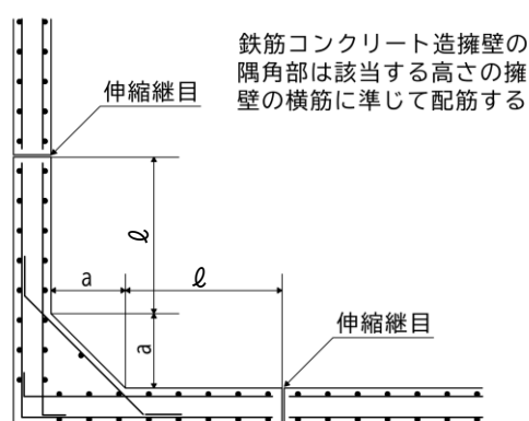
鉄筋コンクリート造擁壁の場合
