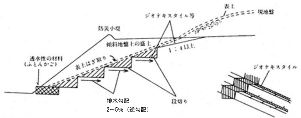
図3-6-2 <湧水が多い場合の排水処理>
