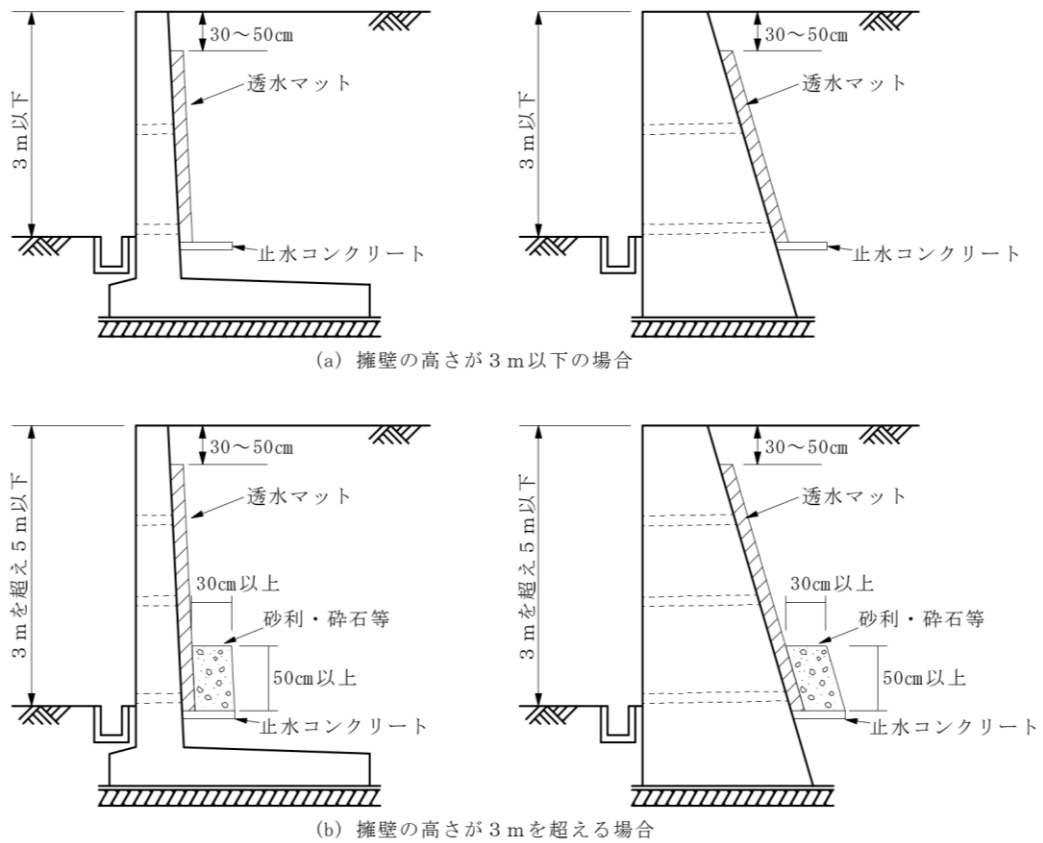
図 5 - 1 透水マット取り付け断面
