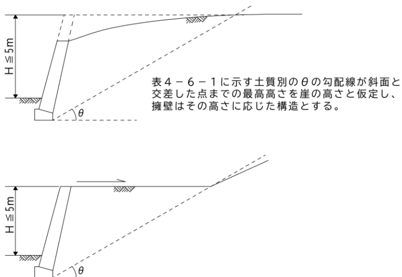
図 4-6-1 &lt;切土部分に設ける練積み造擁壁の場合&gt;
