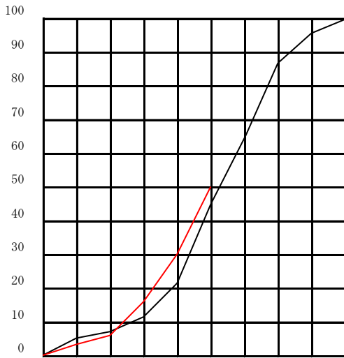
工事進捗率 (%)
