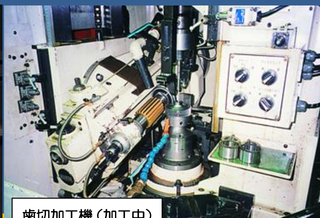
歯切加工機(加工中)
