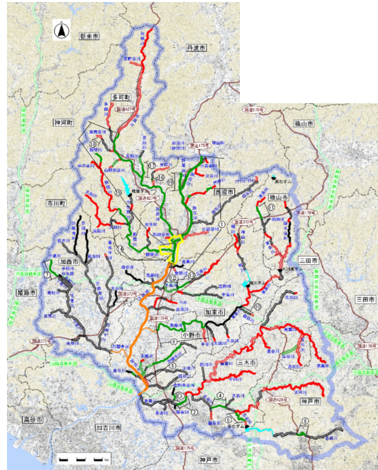
河道改修状況図
