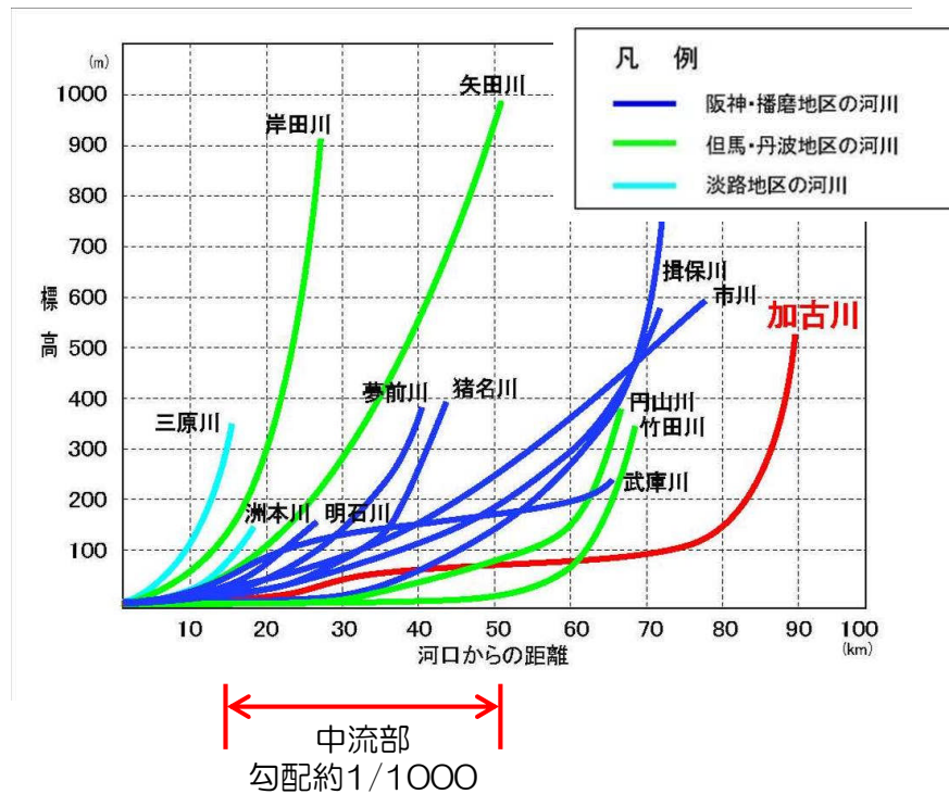
兵庫県下の川の縦断地形（勾配比較）
