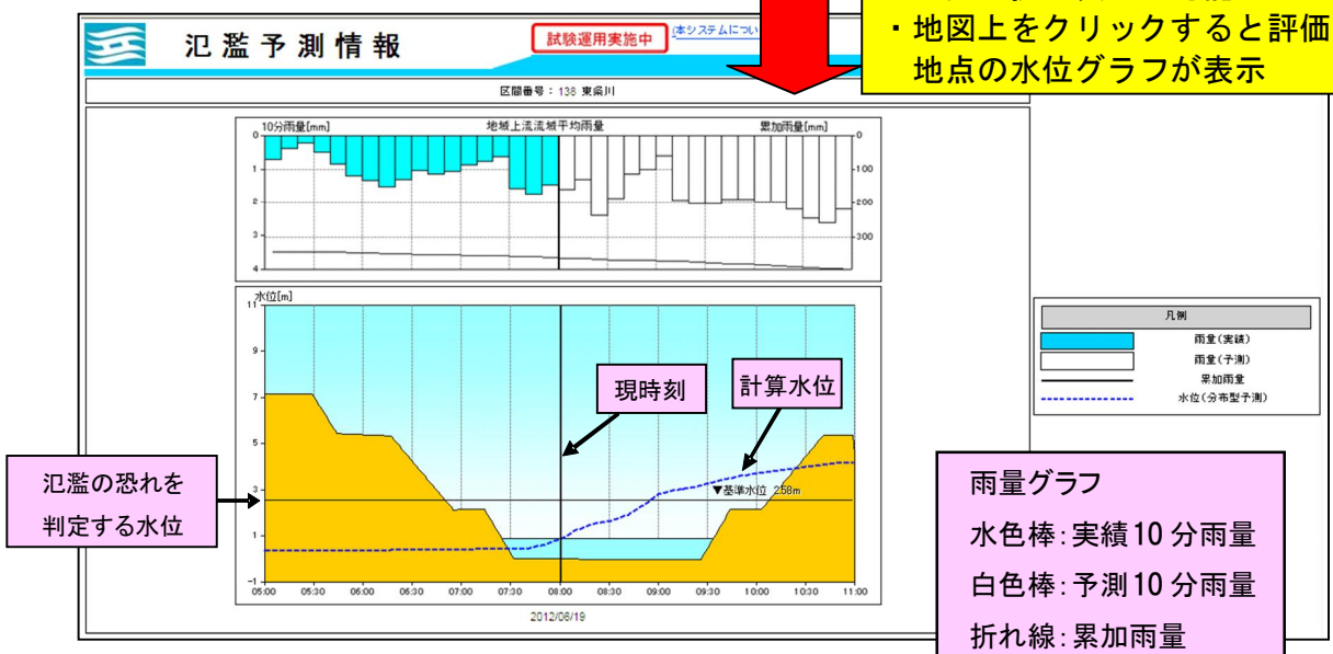
図 44 氾濫予測の例
