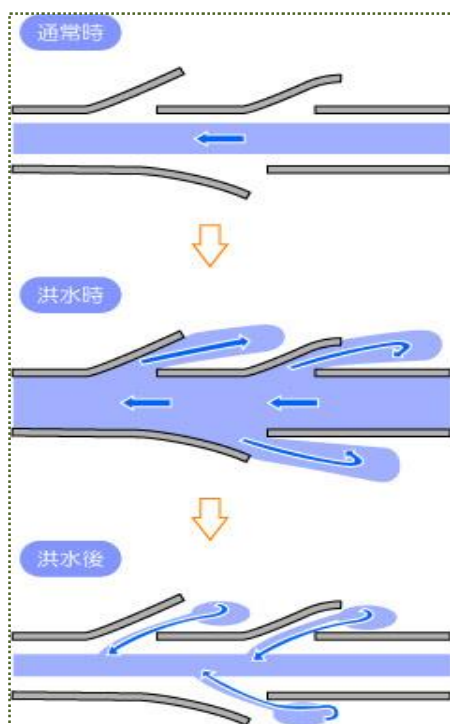
図 35 霞堤のイメージ
