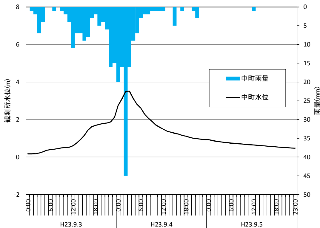
平成23年台風12号洪水 ハイδροグラフ
