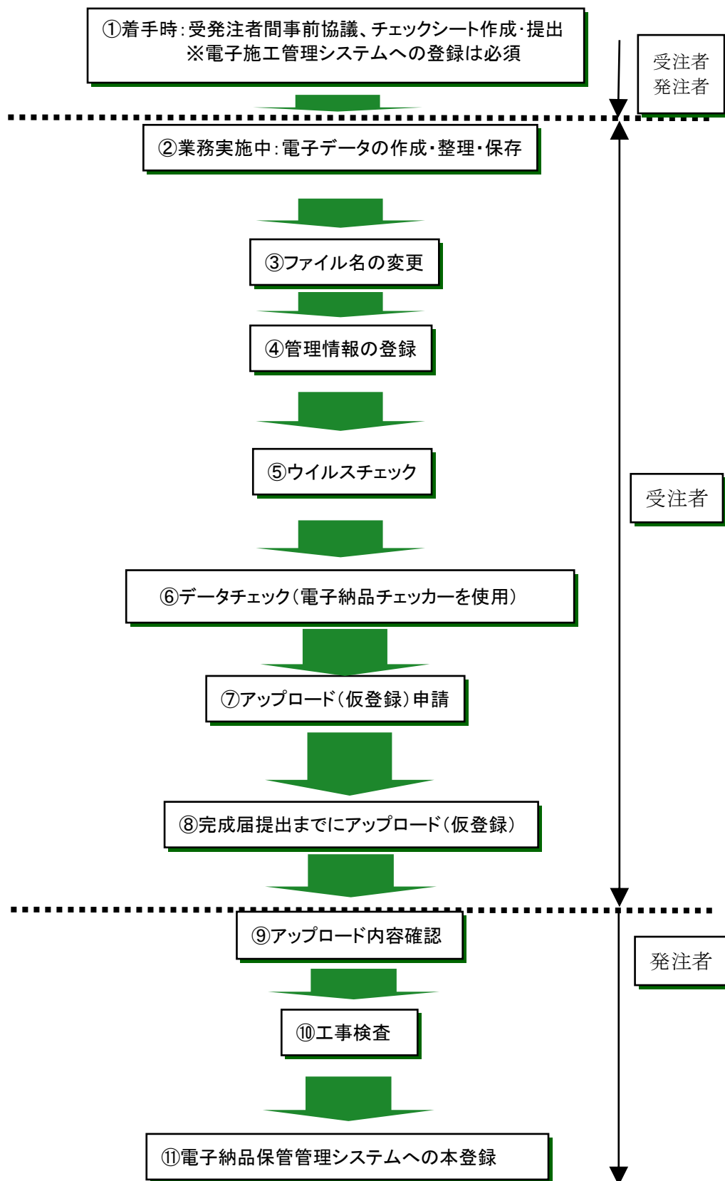
図 2-1 電子成果品の作成手順
