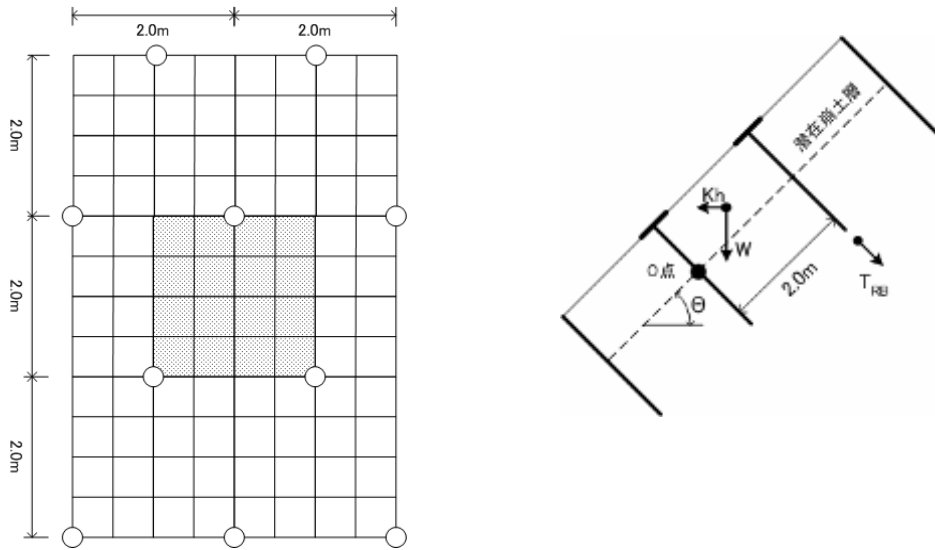
図 4. 3. 14 局所破壊時の土塊モデル
