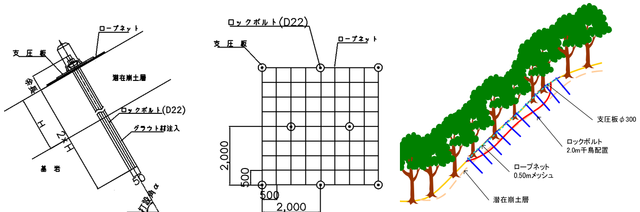
図 1. 3.1 本対策工概要図 (標準的な構造)
