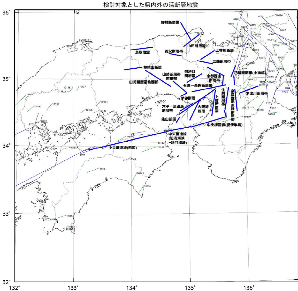
図 4. 3. 3 想定地震の断層モデル 4) (兵庫県地域防災計画から抜粋)
