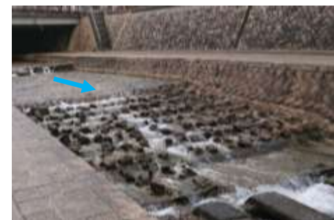
全断面式魚道（粗石付き斜路）の設置 （二）住吉川水系住吉川（神戸市東灘区）
